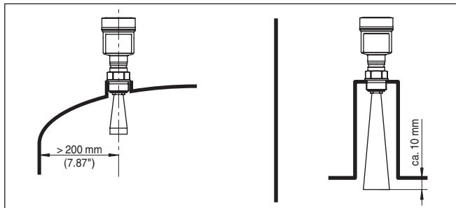
Рис. 5: Расстояние от антенны до стенки емкости/крыши емкости
