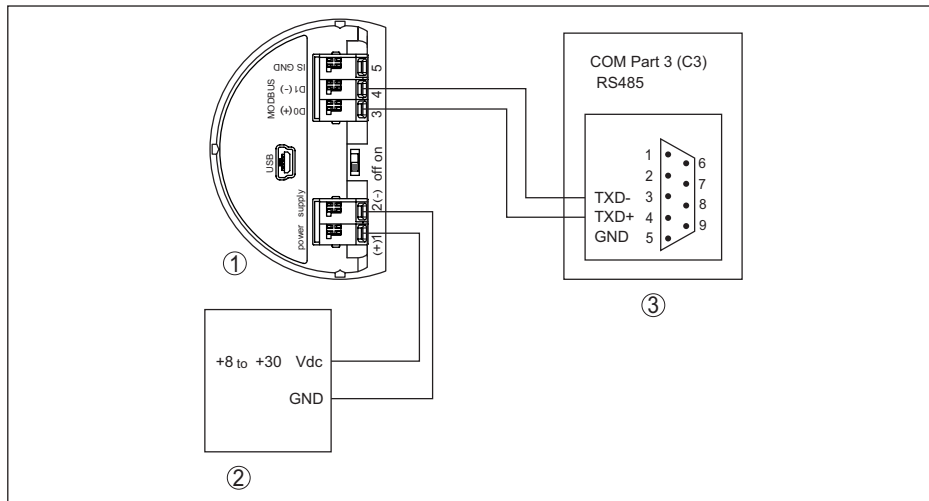
Рис. 50: Подключение VEGAPULS 66 к RTU ScadaPack
