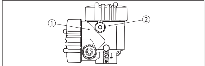
Рис. 16: Позиция отсека подключения (электроника Modbus) и отсека электроники (электроника датчика)
