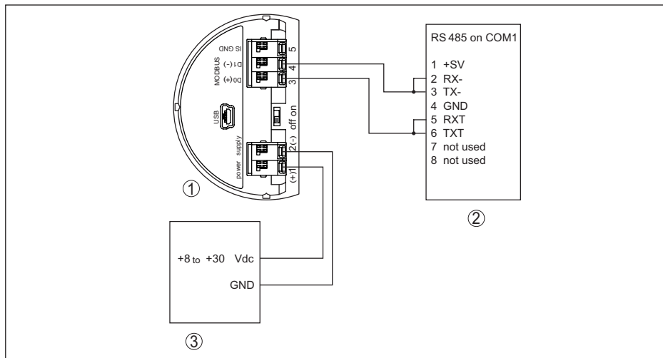
Рис. 49: Подключение VEGAPULS 66 к RTU Bristol ControlWave Micro
