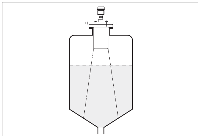
Рис. 5: Монтаж радарного датчика на емкостях с коническим дном
