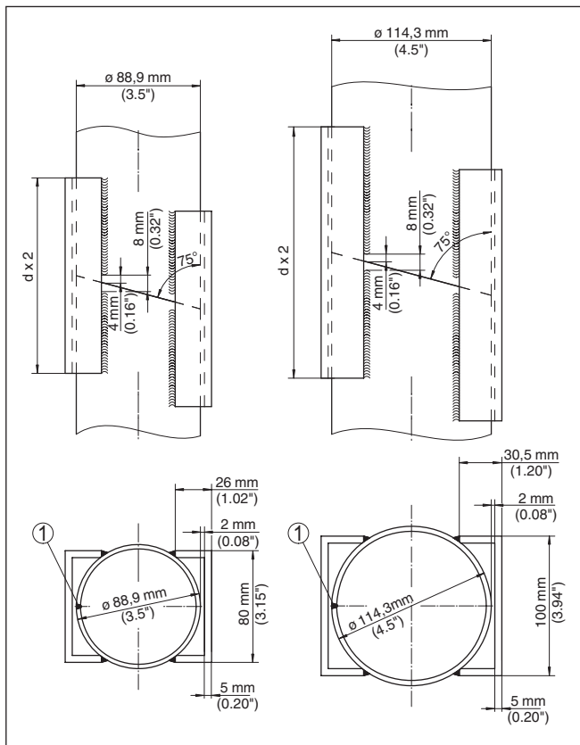
Рис. 12: Сварное соединение при удлинении уравнильной трубы (примеры для различных диаметров)
