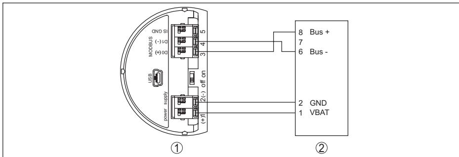
Рис. 47: Подключение VEGAPULS 66 к RTU ABB Total Flow
