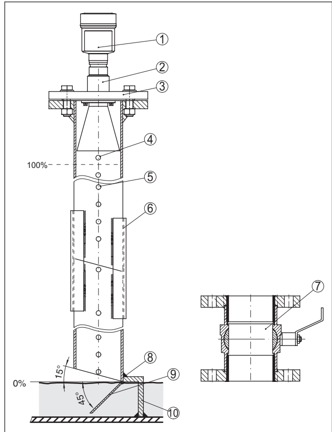
Рис. 11: Монтаж VEGAPULS 66 в уравнильной трубе
