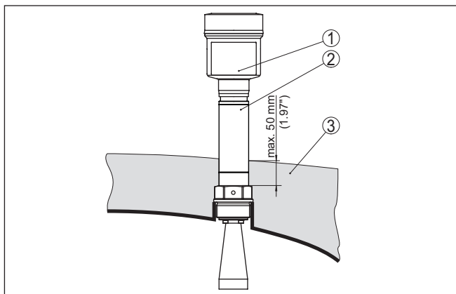
Рис. 14: Монтаж устройства на емкости с термоизоляцией
