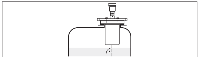
Рис. 8: Ориентация датчика на жидкостях
