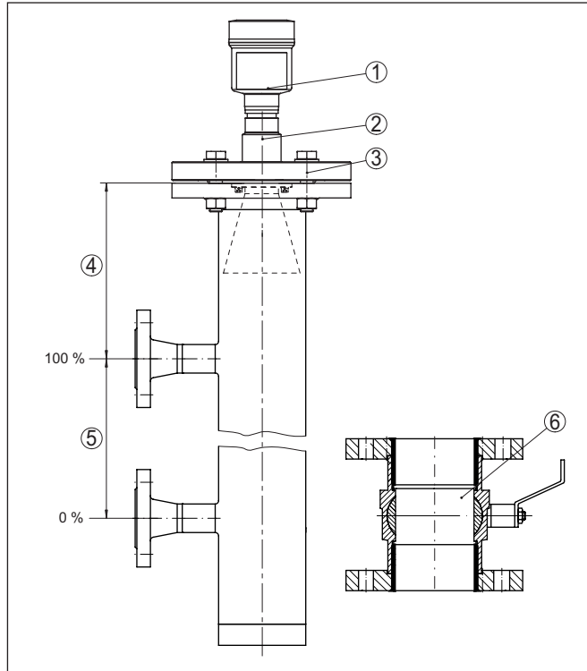
Рис. 13: Монтаж в выносной трубе
