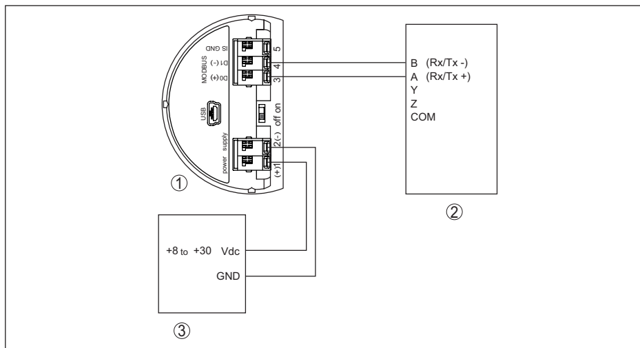
Рис. 46: Подключение VEGAPULS 66 к RTU Fisher ROC 809
