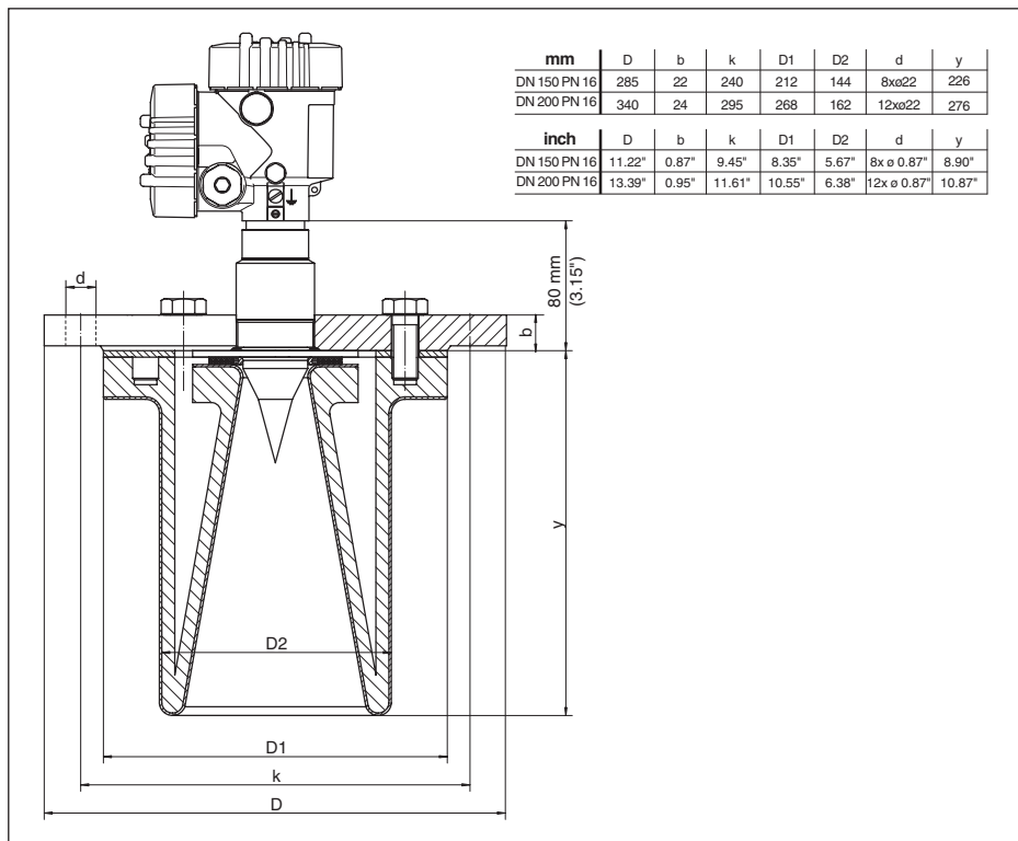
Рис. 52: VEGAPULS 66 с эмалевым покрытием
