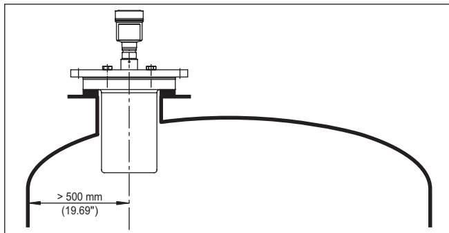
Рис. 4: Монтаж радарного датчика на округлой крыше емкости
