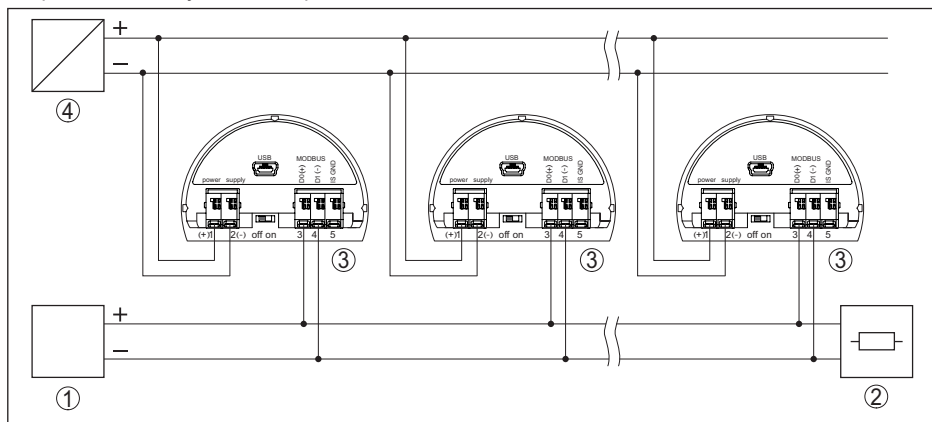
Рис. 45: Архитектура шины Modbus
