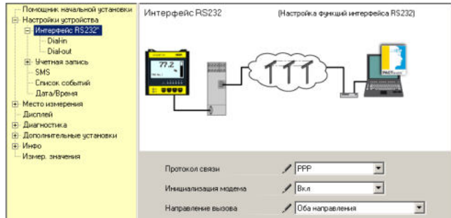
Рис. 8: Конфигурация RS232
