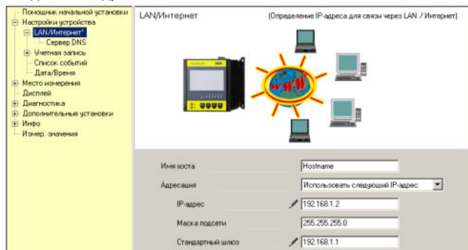
Рис. 17: Присвоение IP-адресов
