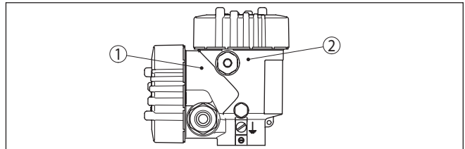
Рис. 7: Позиция отсека подключения (электроника Modbus) и отсека электроники (электроника датчика)
