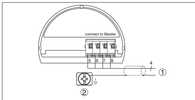
Рис. 4: Схема подключения ведомого датчика VEGABAR 86
