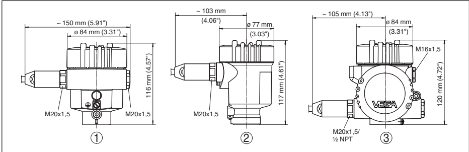
Рис. 29: Корпус в исполнении IP 66/IP 68 (1 bar) - с установленным модулем индикации и настройки корпус выше на 9 mm/0.35 in
