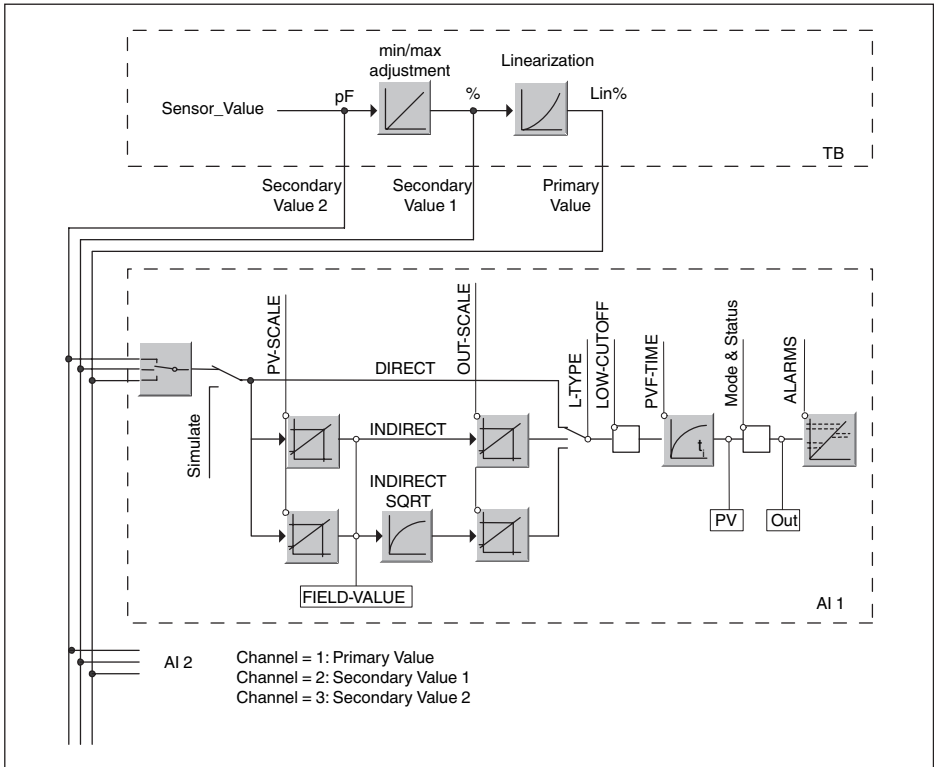
Рис. 26: Обработка измеренных значений VEGACAL 66
