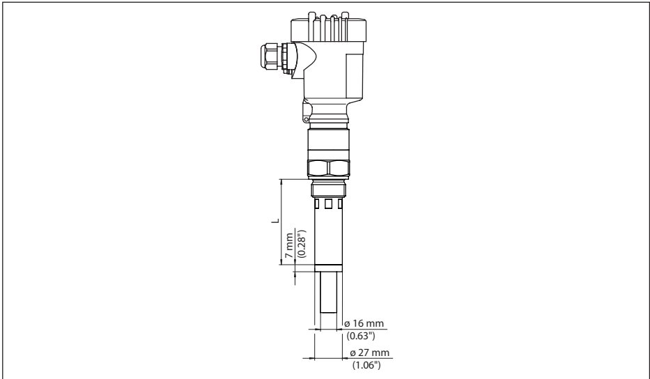
Рис. 31: VEGACAL 66, экранирующая труба (например для защиты от конденсата)
