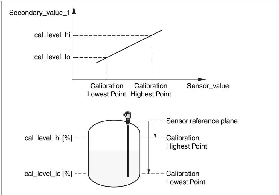
Рис. 27: Установка VEGACAL 66
