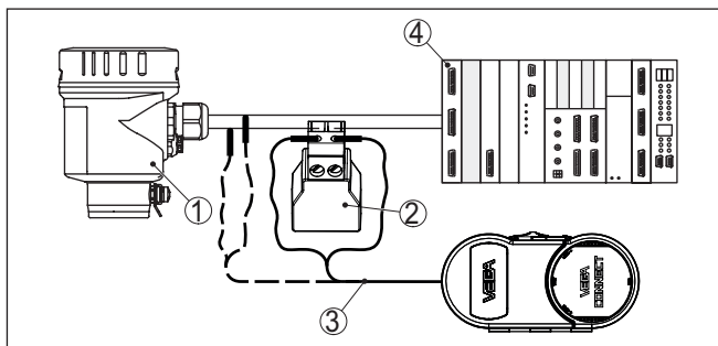
Рис. 44: Подключение ПК к сигнальному кабелю через HART
