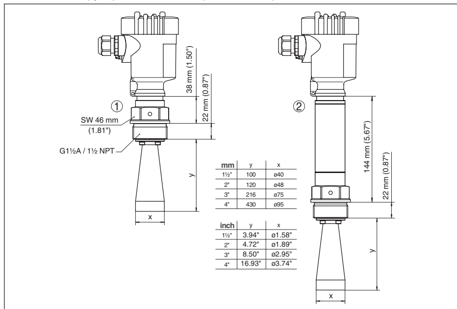
Рис. 63: VEGAPULS 68 с рупорной антенной и резьбовым присоединением
