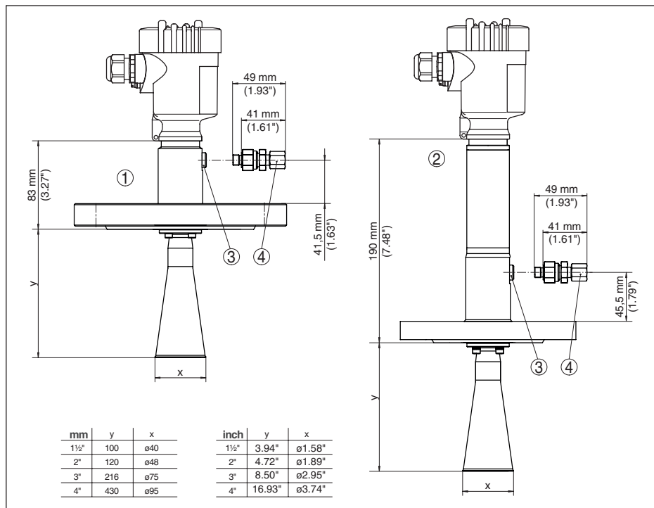
Рис. 65: VEGAPULS 68, с рупорной антенной и фланцевым присоединением, со входом для подключения продувки
