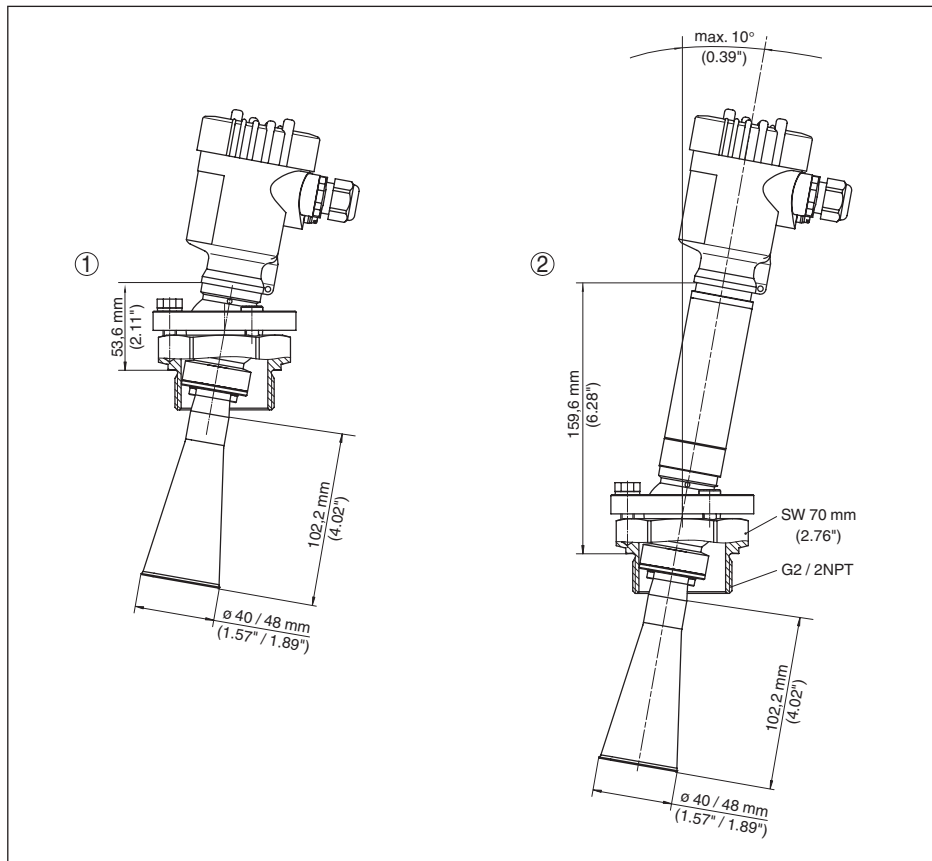
Рис. 68: VEGAPULS 68, рупорная антенна и поворотный держатель, резьбовое присоединение
