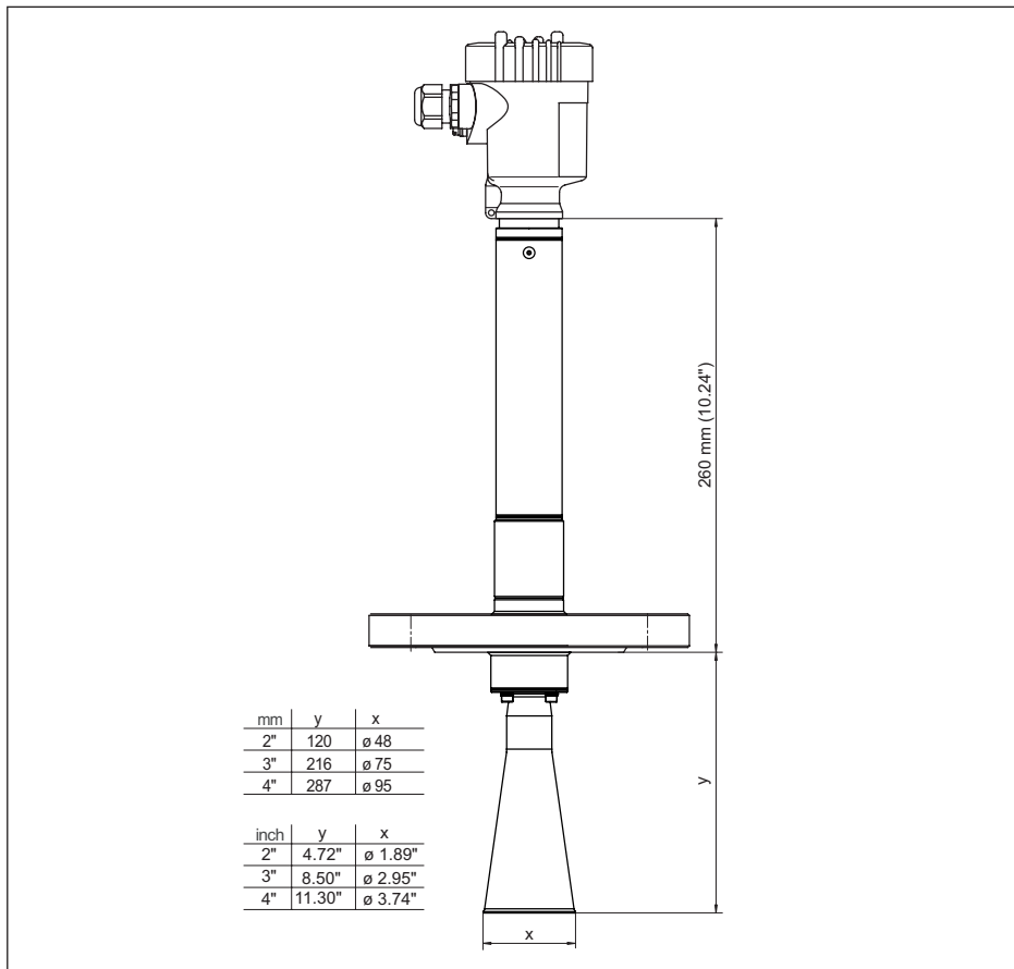
Рис. 66: VEGAPULS 68, с рупорной антенной и фланцевым присоединением, с температурной вставкой до 450 °С
