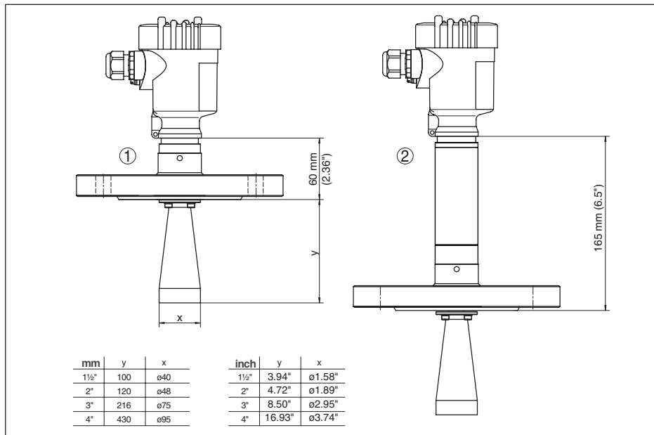
Рис. 64: VEGAPULS 68, с рупорной антенной и фланцевым присоединением
