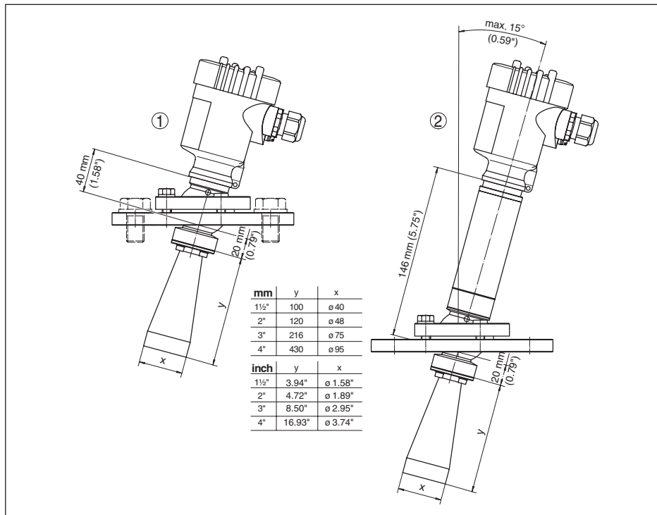
Рис. 67: VEGAPULS 68, с рупорной антенной и поворотным креплением
