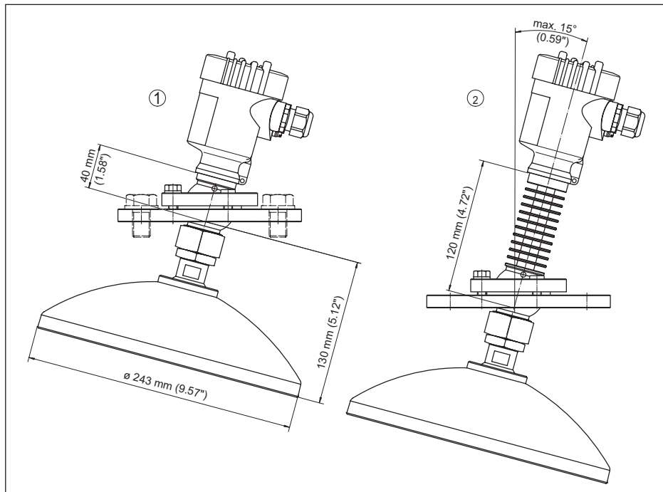
Рис. 69: VEGAPULS 68, с параболической антенной и поворотным креплением
