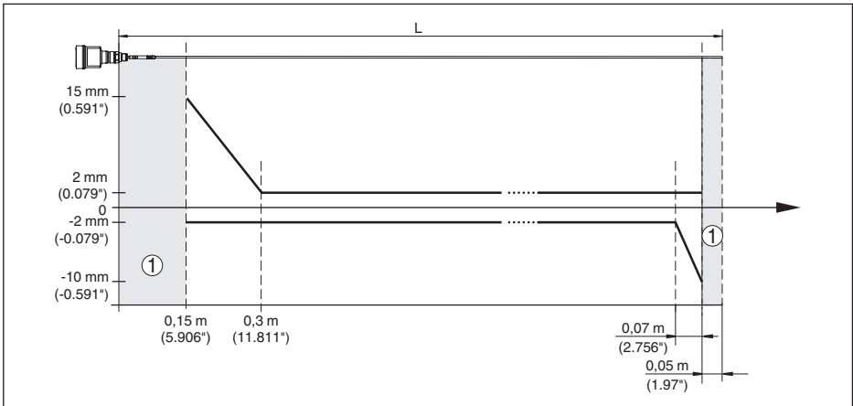
Рис. 51: Погрешность измерения VEGAFLEX 81 в стержневом исполнении (среда - масло)
