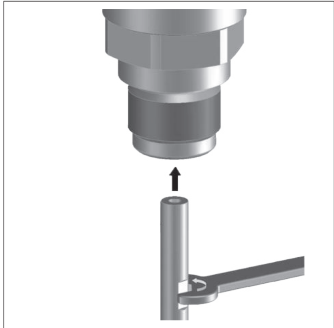
Рис. 47: Замена измерительного троса или стержня
