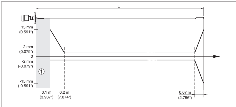
Рис. 55: Погрешность измерения VEGAFLEX 81 в тросовом исполнении \varnothing 4 \text{ mm}/0.157 \text{ in} , с покрытием PFA (среда - вода)
