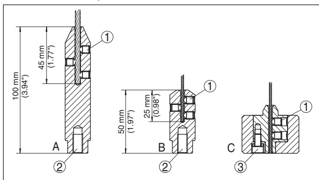
Рис. 48: Укорачивание измерительного троса
