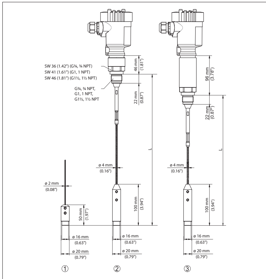
Рис. 73: VEGAFLEX 81, резьбовое исполнение с натяжным грузом (все натяжные грузы с резьбой M8 для рым-болта)
