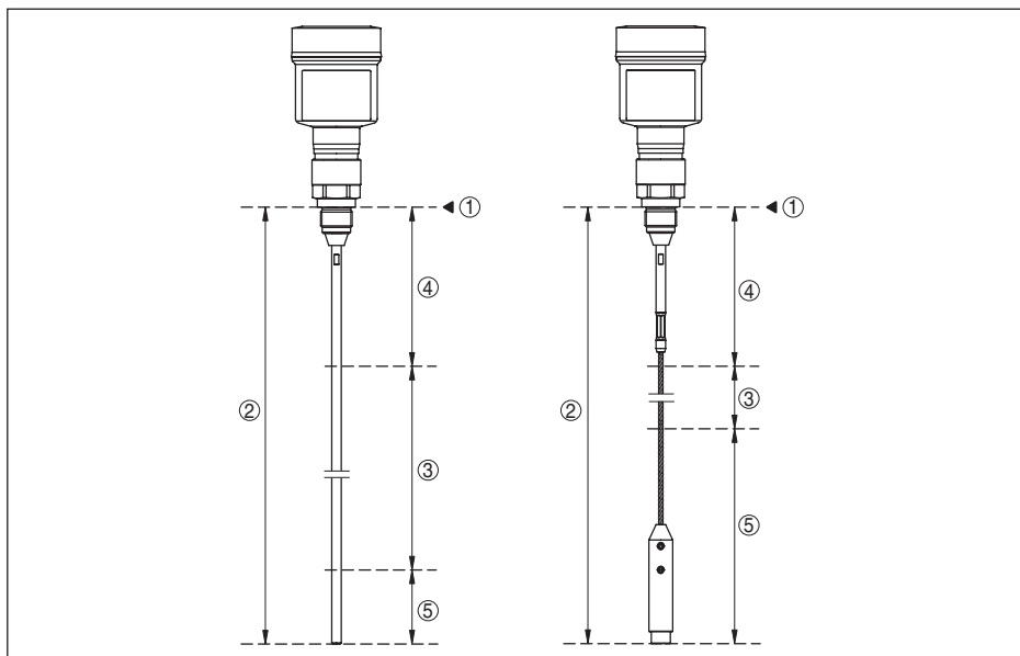
Рис. 49: Диапазоны измерения - VEGAFLEX 81
