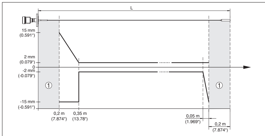
Рис. 56: Погрешность измерения VEGAFLEX 81 в тросовом исполнении \varnothing 4 \text{ мм}/0.157 \text{ in} , с покрытием PFA (среда - масло)
