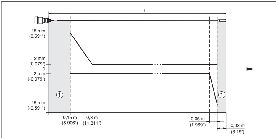
Рис. 53: Погрешность измерения VEGAFLEX 81 в тросовом исполнении \varnothing 2 mm/0.079 in (среда - масло)
