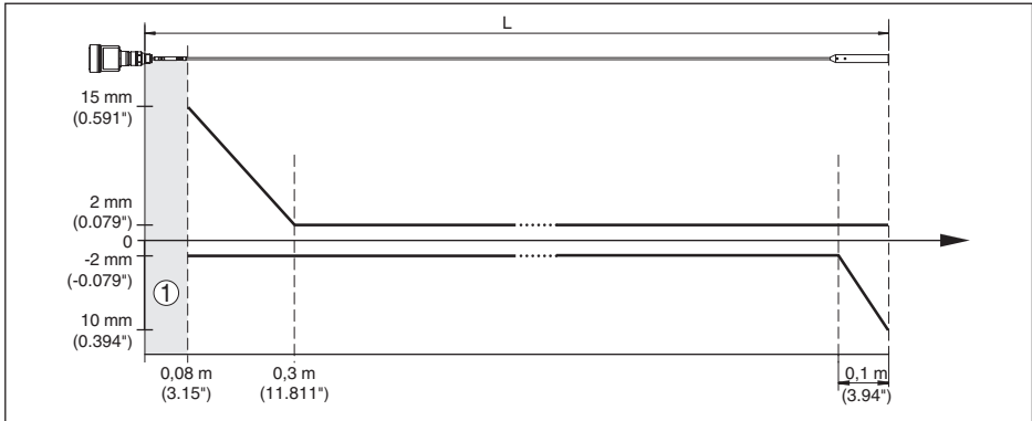
Рис. 52: Погрешность измерения VEGAFLEX 81 в тросовом исполнении (среда - вода)
