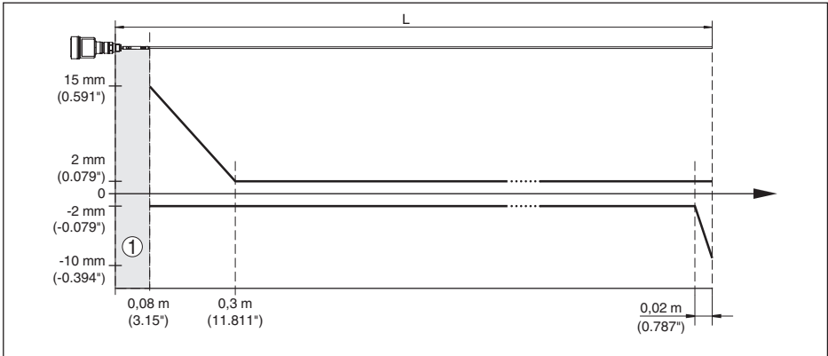
Рис. 50: Погрешность измерения VEGAFLEX 81 в стержневом исполнении (среда - вода)
