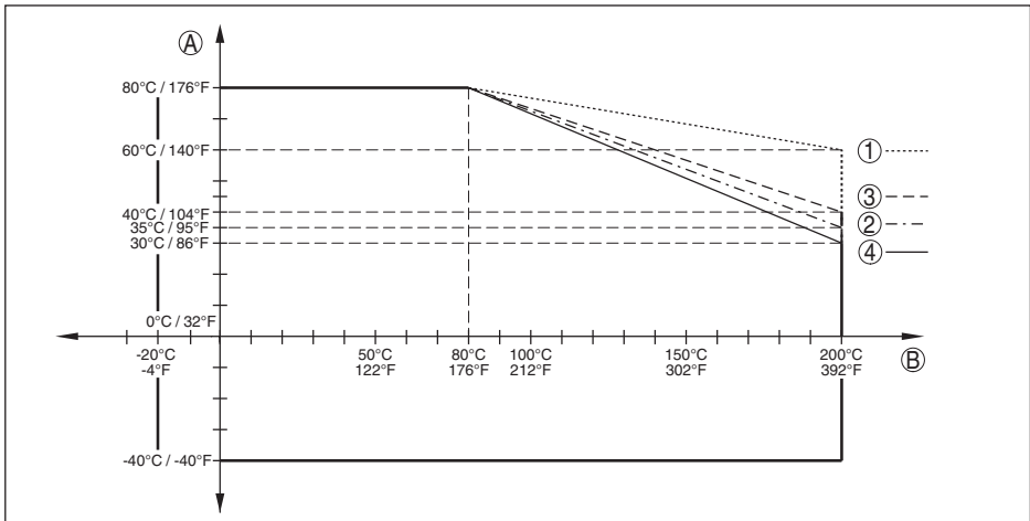
Рис. 58: Температура окружающей среды - температура процесса, исполнение с температурной вставкой
