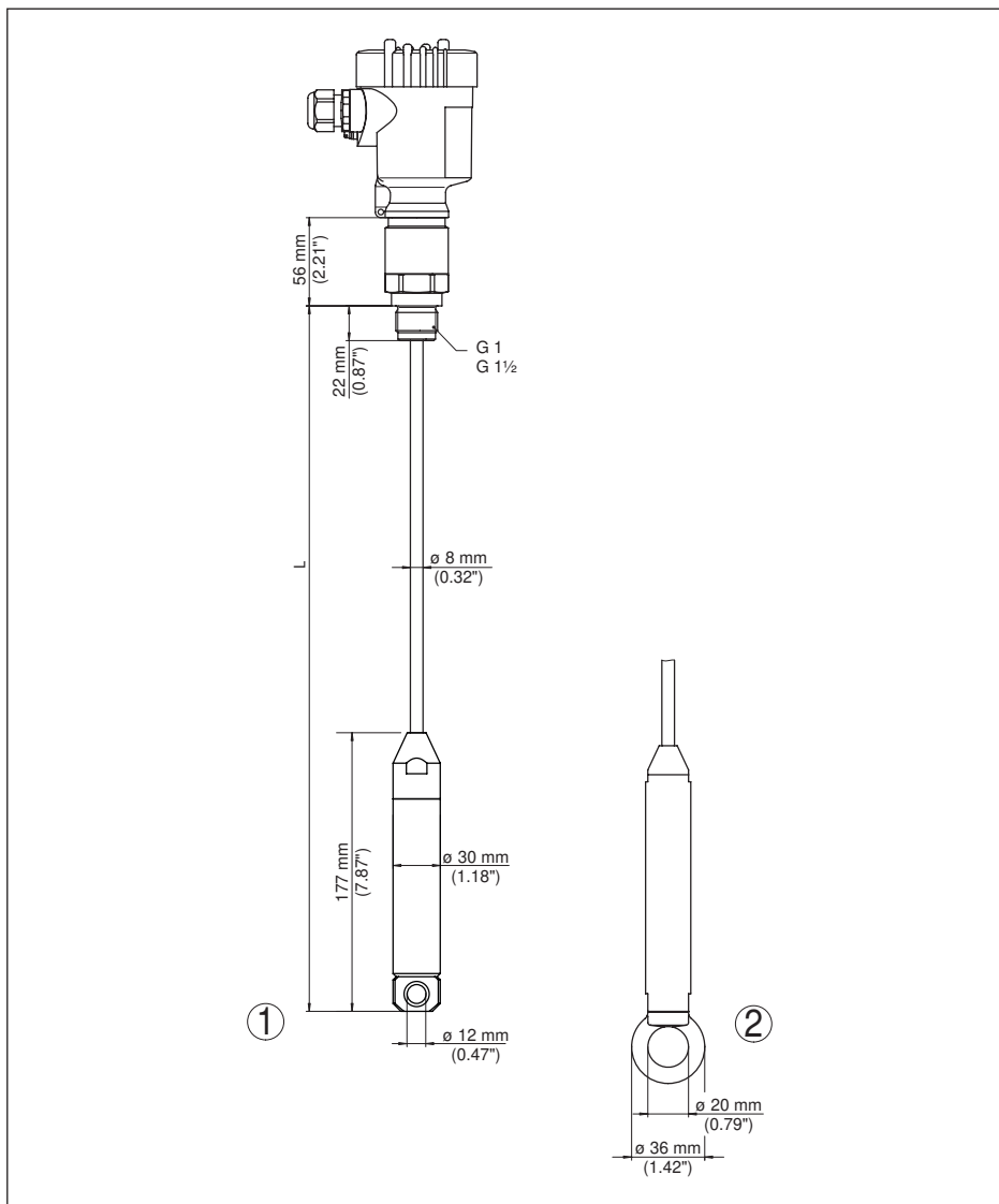
Рис. 31: VEGACAL 66, Резьбовое исполнение G1 (ISO 228 T1)
