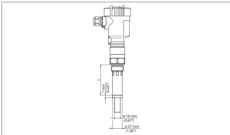
Рис. 32: VEGACAL 66, экранирующая труба (например для защиты от конденсата)
