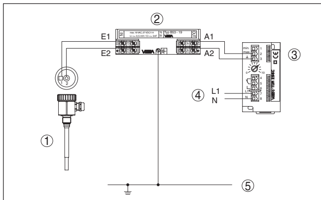
Рис. 8: Схема подключения V53-19 с кондуктивным однострержневым измерительным зондом
