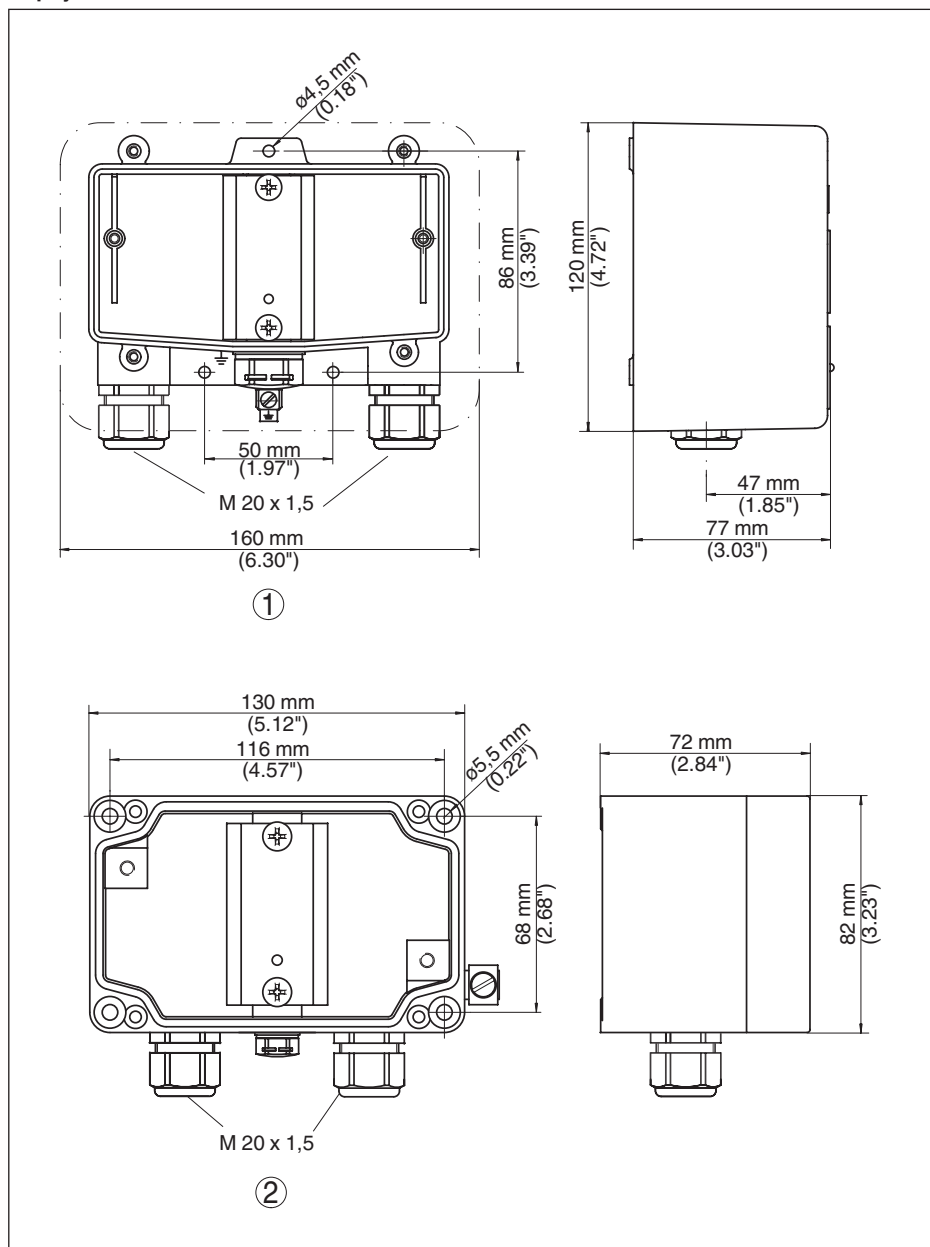
Рис. 11: Размеры V53-19
