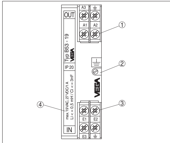
Рис. 1: Конструкция устройства V53-19
