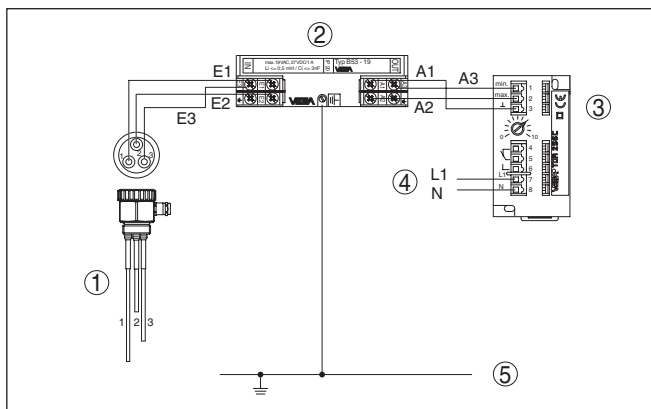
Рис. 9: Схема подключения V53-19 с кондуктивным трехстрержневым измерительным зондом
