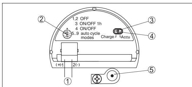
Рис. 3: Отсек питания
