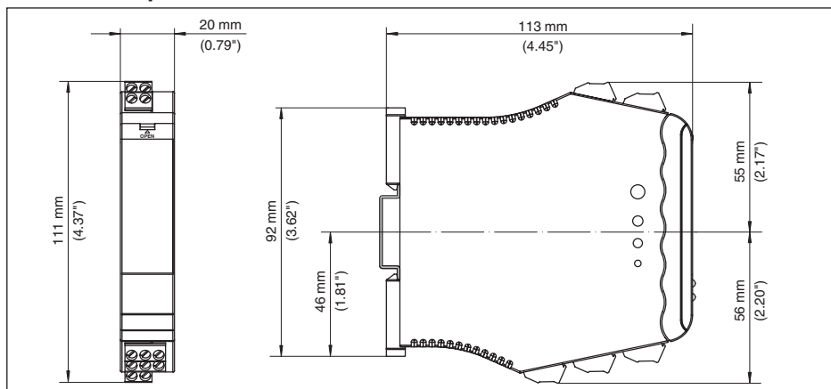
Рис. 54: Размеры VEGATOR 112
