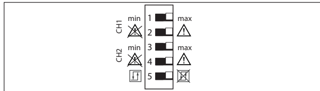
Рис. 3: DIL-переключатель VEGATOR 112
