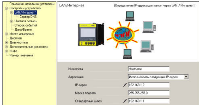
Рис. 19: Присвоение IP-адресов
