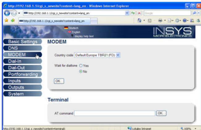
Рис. 25: Конфигурация модема
