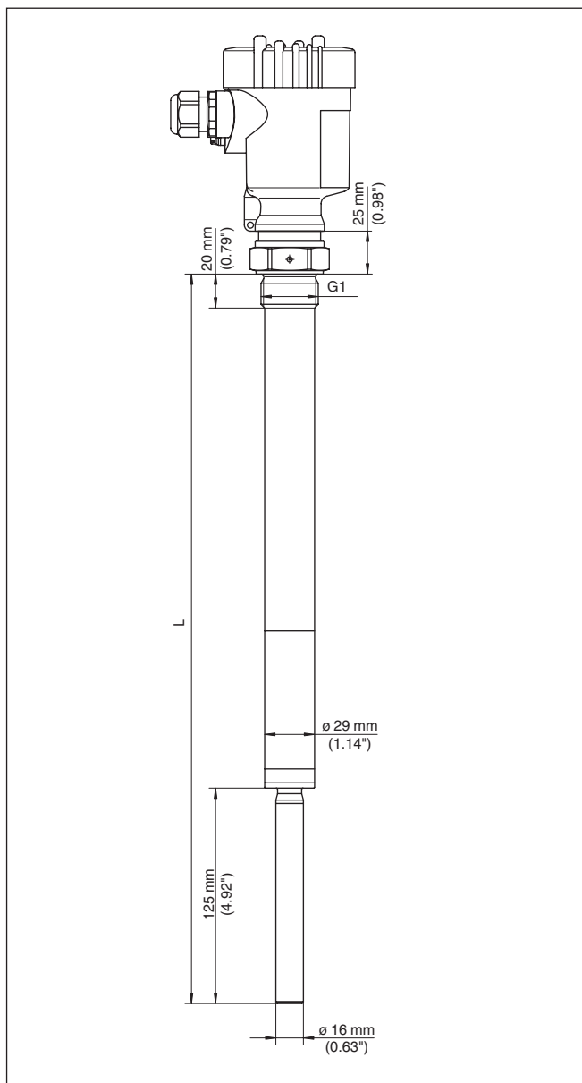
Рис. 34: VEGAVIB 63, резьбовое исполнение G1 A (DIN ISO 228/1)
