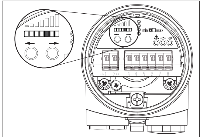
Рис. 42: Индикаторная полоска - установка для продуктов с малым демпфированием сигнала
