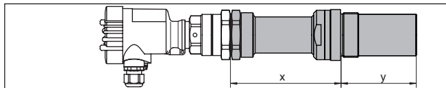
Рис. 5: VEGAMIP 62 с монтажным адаптером для высоких температур с тубусом -40 ... +450 °C (-40 ... +842 °F)
