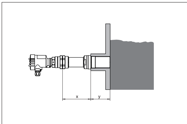
Рис. 15: Монтажный адаптер для высоких температур -40 \dots +450 \text{ }^\circ\text{C} ( -40 \dots +842 \text{ }^\circ\text{F} ) с тубусом для монтажа заподлицо в длинной патрубке
