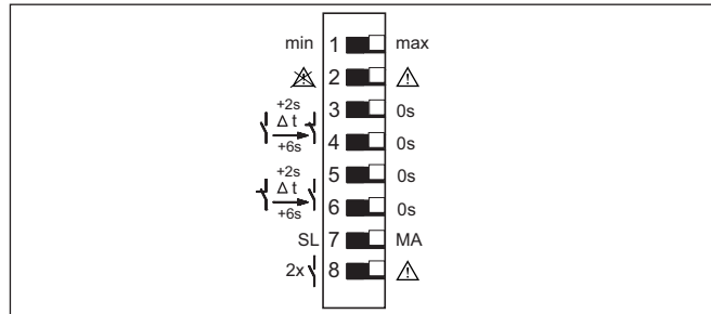
Рис. 3: DIL-переключатель VEGATOR 131
