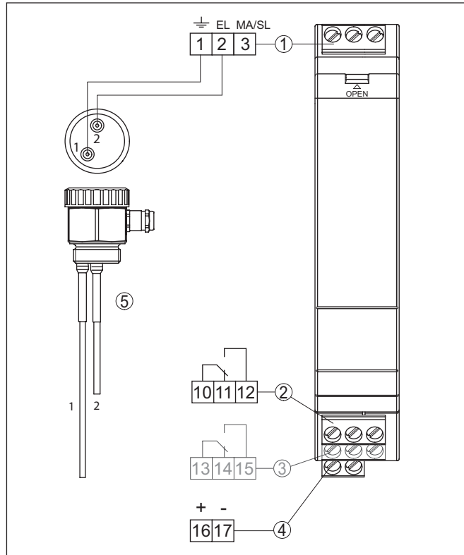
Рис. 1: Схема подключения VEGATOR 131
