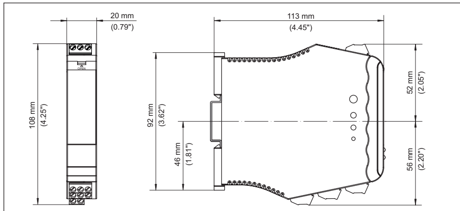
Рис. 21: Размеры VEGATOR 131
