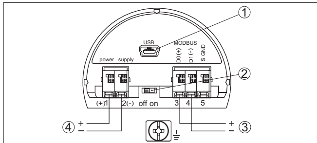
Рис. 16: Отсек подключения
