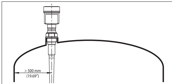
Рис. 5: Монтаж радарного датчика на округлой крыше емкости
