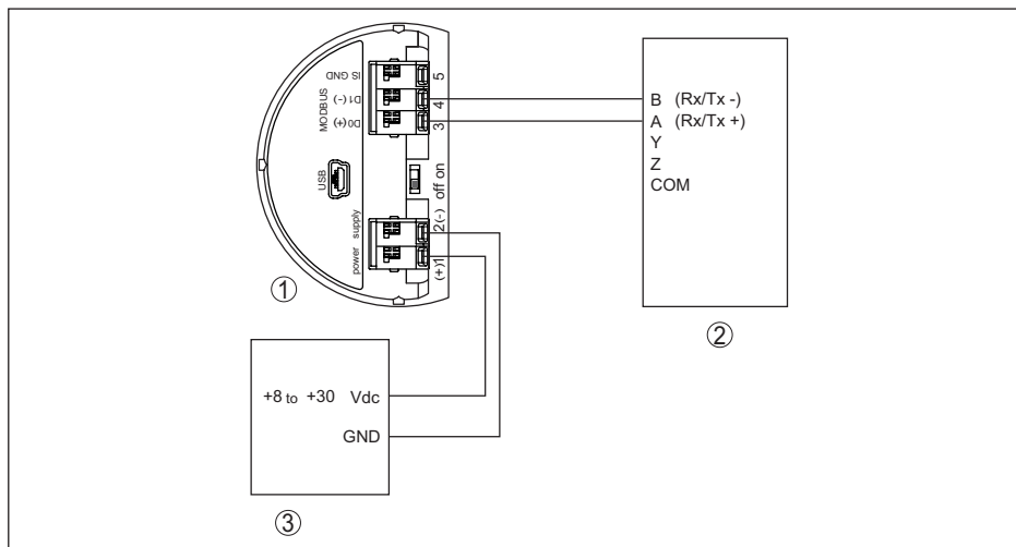
Рис. 30: Подключение VEGAPULS 65 к RTU Fisher ROC 809
