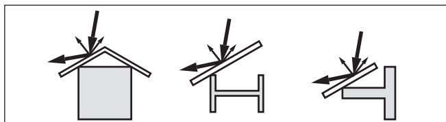
Рис. 10: Отражатели над конструкциями в емкости
