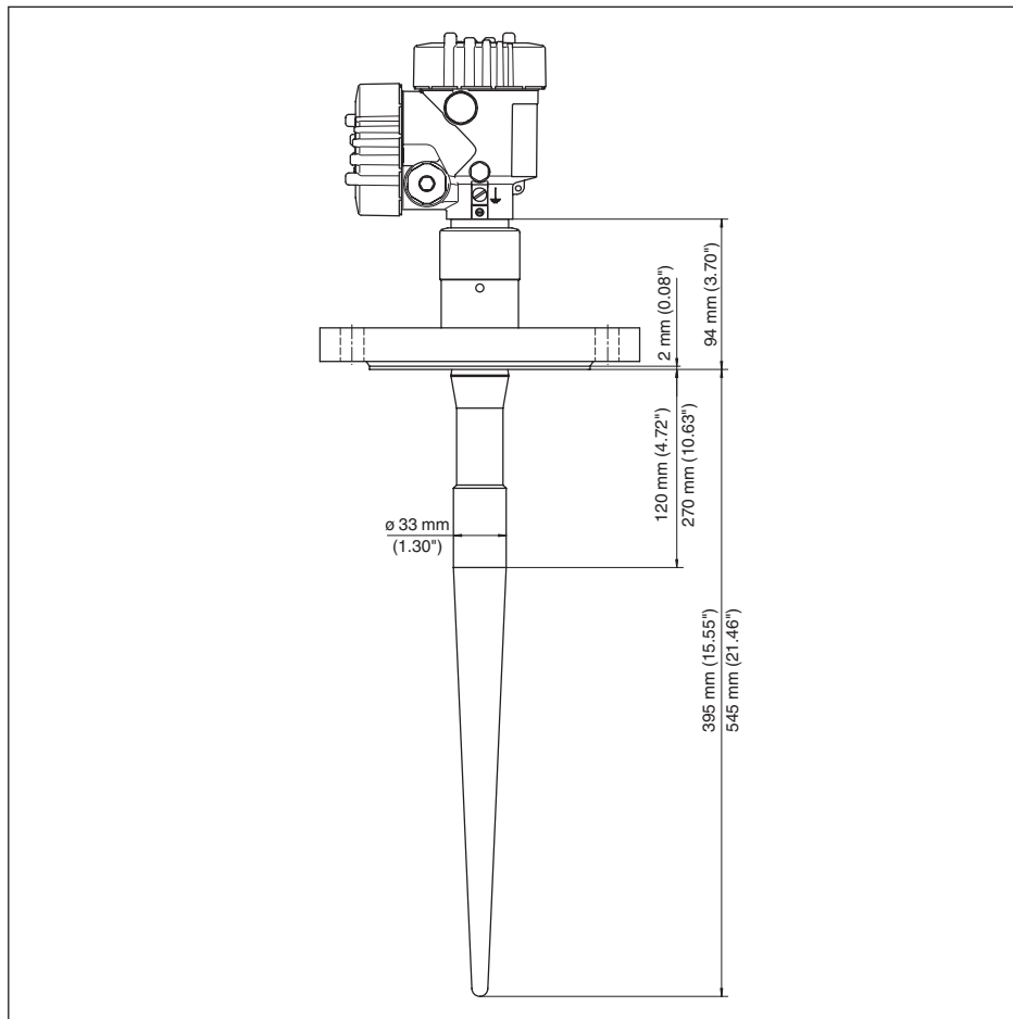
Рис. 37: VEGAPULS 65 во фланцевом исполнении для патрубков высотой 100 мм (неактивная длина 120 мм) или 250 мм (неактивная длина 270 мм)
