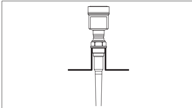
Рис. 8: Рекомендуемая высота монтажного патрубка
