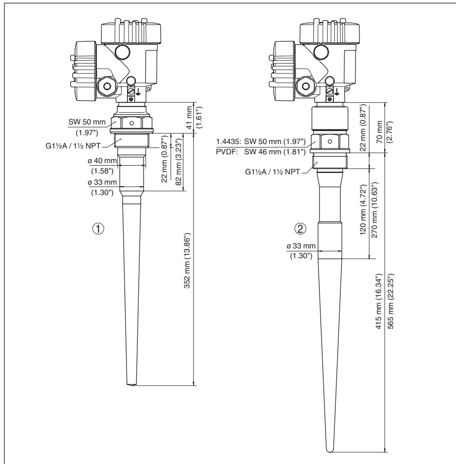
Рис. 36: VEGAPULS 65, резьбовое исполнение
