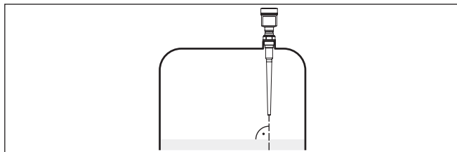
Рис. 9: Ориентация датчика на жидкостях
