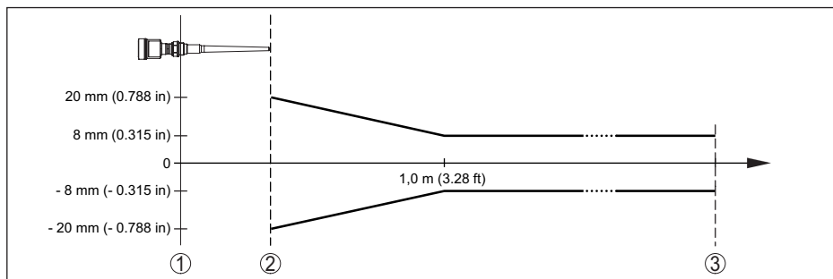
Рис. 28: Погрешность измерения при эталонных условиях
