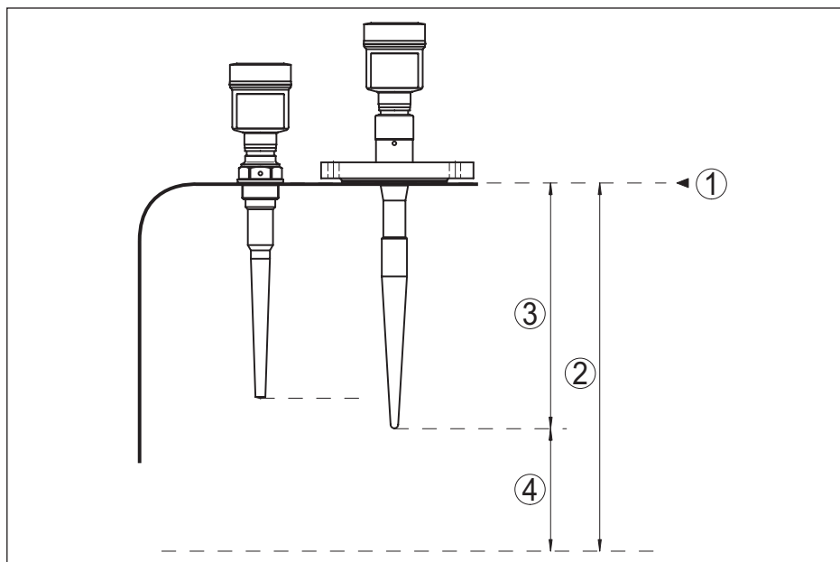
Рис. 27: Данные для входной величины
