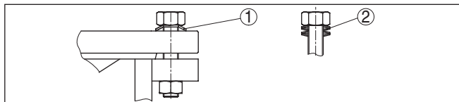
Рис. 3: Использование дисковых пружин
