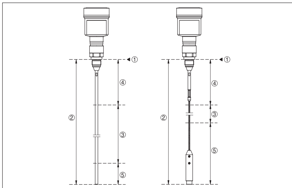
Рис. 45: Диапазоны измерения - VEGAFLEX 81
