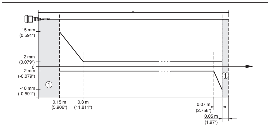
Рис. 47: Погрешность измерения VEGAFLEX 81 в стержневом исполнении (среда - масло)
