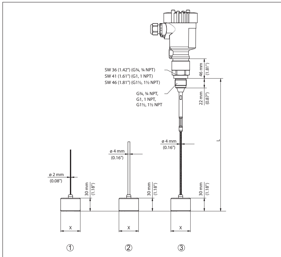
Рис. 61: VEGAFLEX 81, резьбовое исполнение
