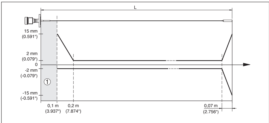
Рис. 51: Погрешность измерения VEGAFLEX 81 в тросовом исполнении \varnothing 4 \text{ mm}/0.157 \text{ in} , с покрытием PFA (среда - вода)
