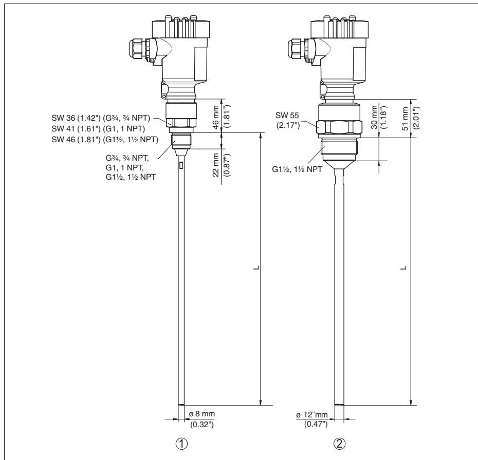
Рис. 62: VEGAFLEX 81, резьбовое исполнение
