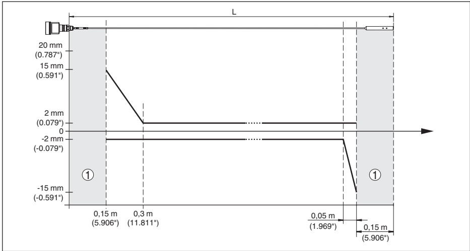
Рис. 50: Погрешность измерения VEGAFLEX 81 в тросовом исполнении \varnothing 4 \text{ mm}/0.157 \text{ in} (среда - масло)
