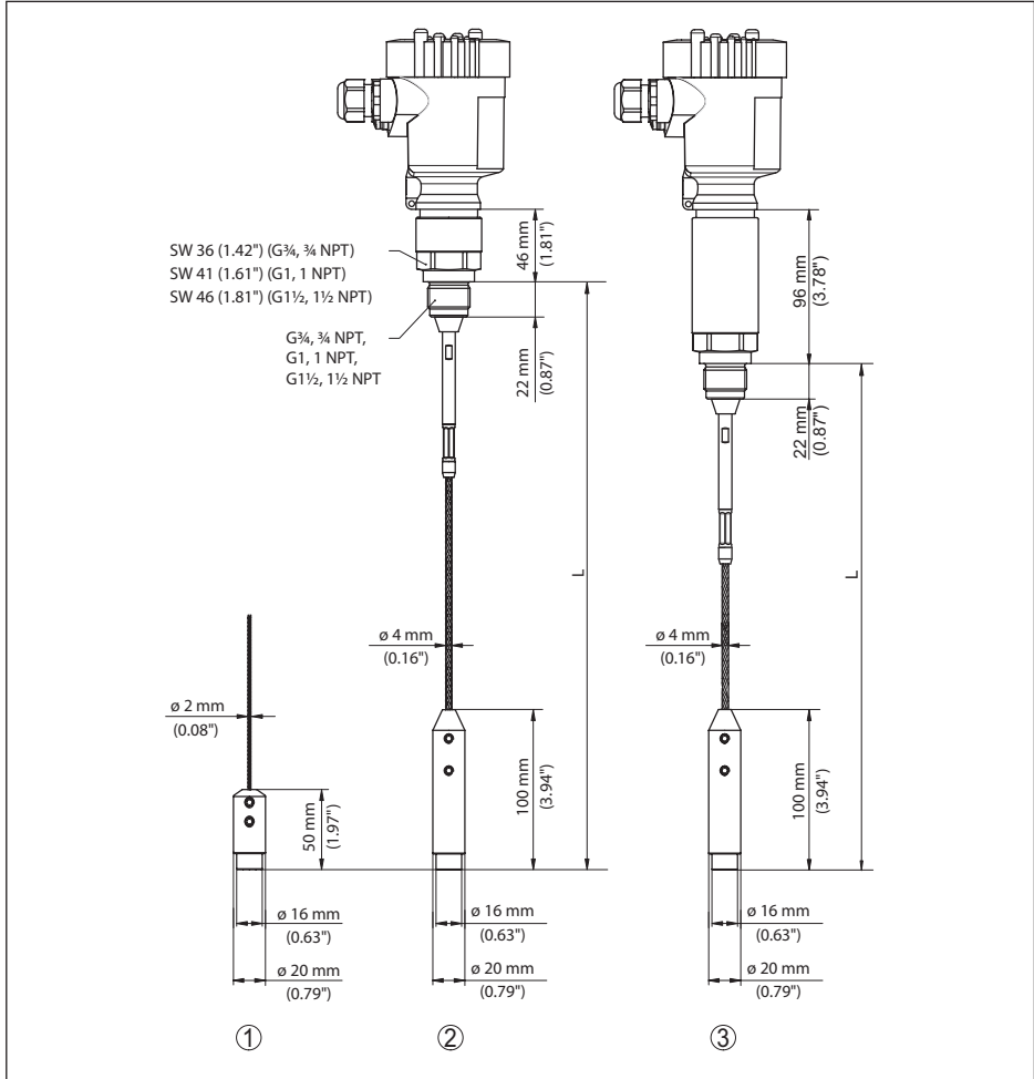
Рис. 60: VEGAFLEX 81, резьбовое исполнение с натяжным грузом (все натяжные грузы с резьбой M8 для рым-болта)
