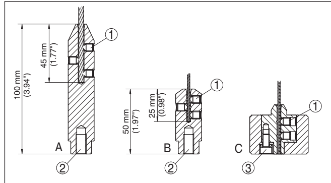
Рис. 44: Укорачивание измерительного троса
