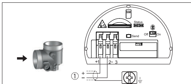
Рис. 18: Отсек подключения - модуль PLICSMOBILE 81
