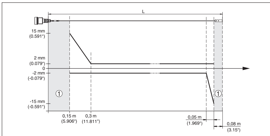
Рис. 49: Погрешность измерения VEGAFLEX 81 в тросовом исполнении \varnothing 2 \text{ mm}/0.079 \text{ in} (среда - масло)
