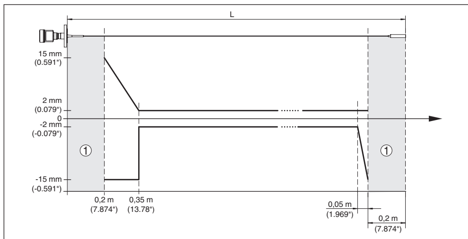
Рис. 52: Погрешность измерения VEGAFLEX 81 в тросовом исполнении \varnothing 4 мм/0.157 in, с покрытием PFA (среда - масло)
