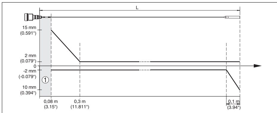
Рис. 48: Погрешность измерения VEGAFLEX 81 в тросовом исполнении (среда - вода)
