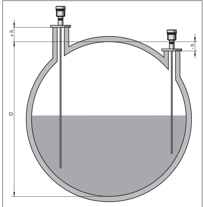
Рис. 28: Высота емкости и значение коррекции патрубка
