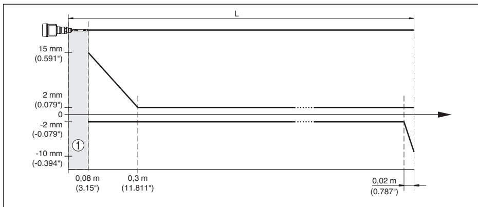
Рис. 46: Погрешность измерения VEGAFLEX 81 в стержневом исполнении (среда - вода)
