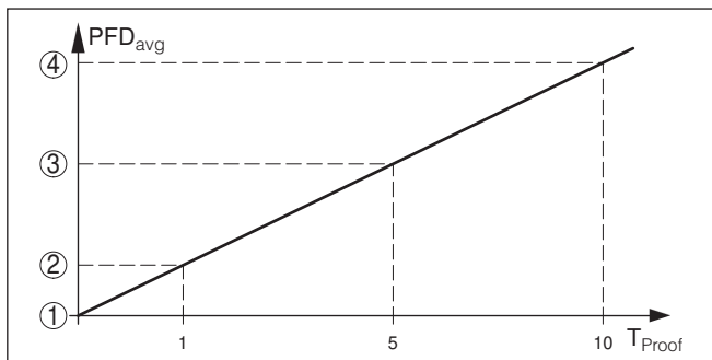
Рис. 1: Изменение PFD_{avg} во времени (числовые значения см. в таблицах выше)
