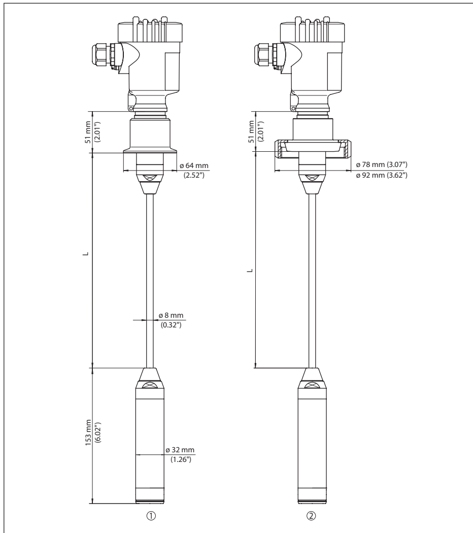
Рис. 33: VEGABAR 86, гигиенические типы присоединения
