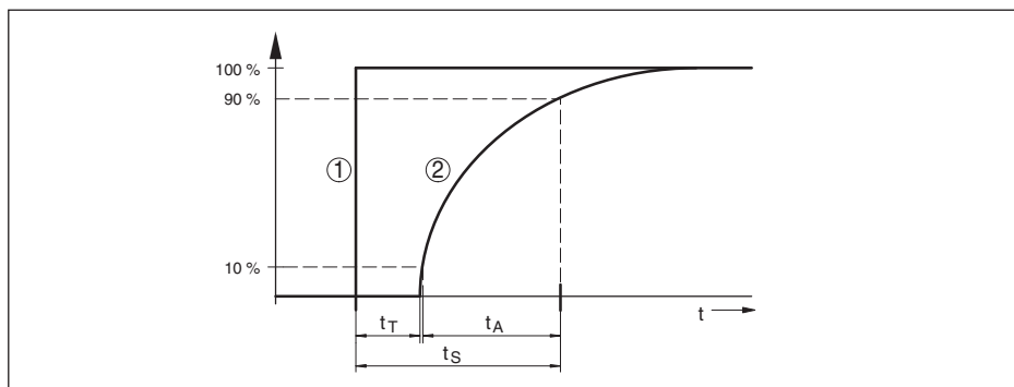
Рис. 23: Состояние при скачкообразном изменении параметров процесса. t_T : время нечувствительности; t_A : время нарастания; t_S : время реакции на скачкообразное изменение
