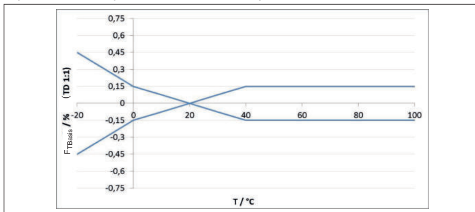
Рис. 24: Базовая температурная погрешность F_{TBasis} при TD 1 : 1
