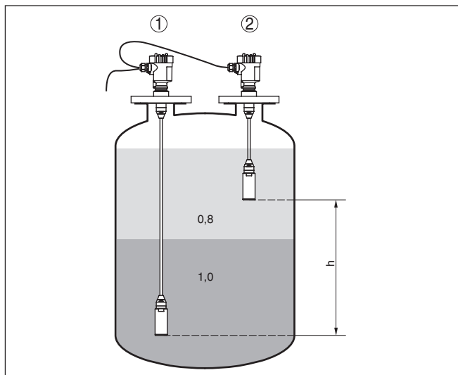
Рис. 10: Измерительная схема для измерения межфазного уровня, h = расстояние между двумя точками измерения
