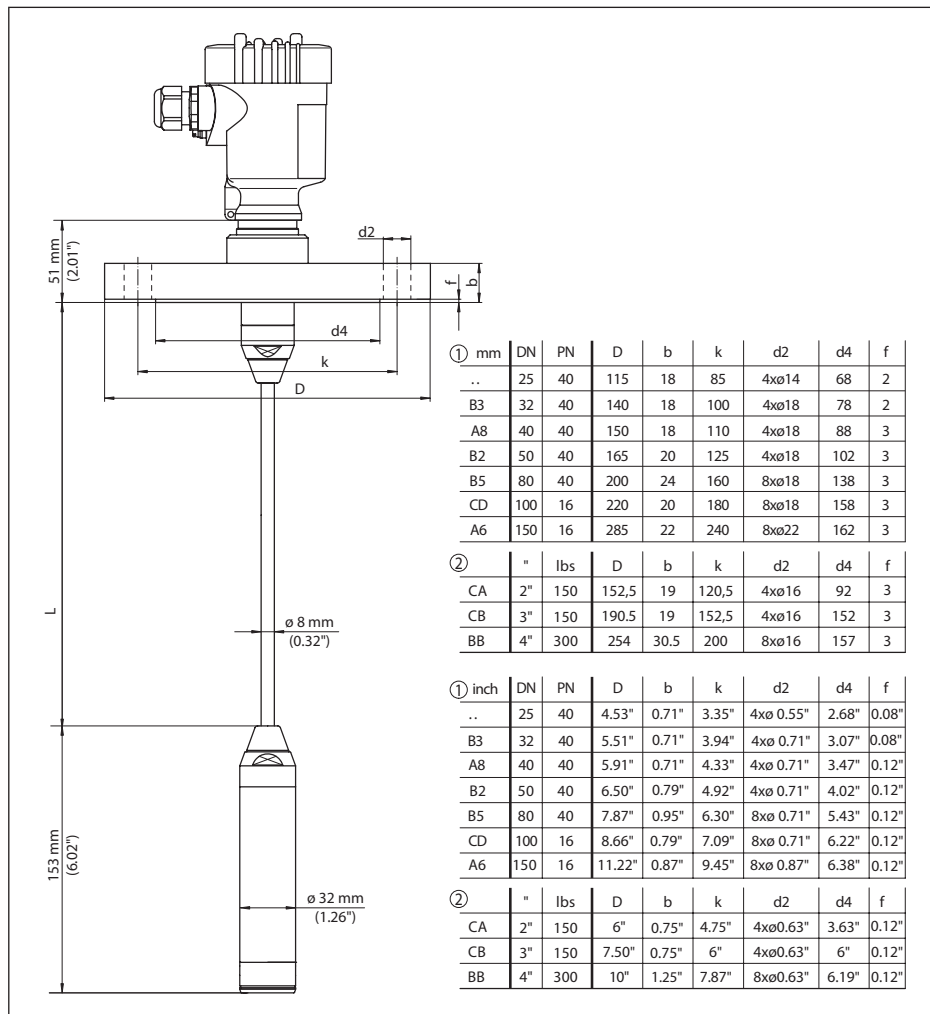
Рис. 32: VEGABAR 86, фланцевое присоединение (пример с чувствительным элементом 32 мм)
