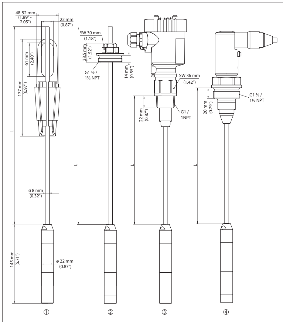
Рис. 29: VEGABAR 86 - чувствительный элемент 22 мм
