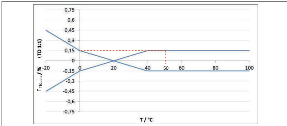
Рис. 25: Определение базовой температурной погрешности для примера выше: F_{\text{T Basis}} = 0,15 \%
