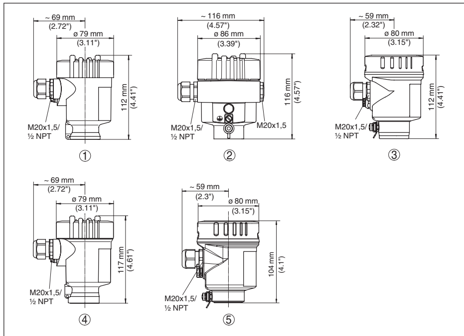
Рис. 27: Исполнения корпуса со степенью защиты IP 66/IP 67 и IP 66/IP 68 (0,2 bar)
