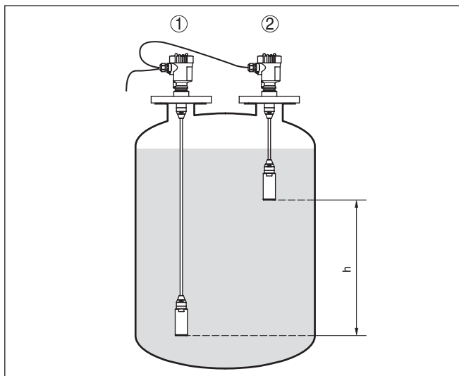
Рис. 11: Измерительная схема для измерения плотности, h = расстояние между двумя точками измерения
