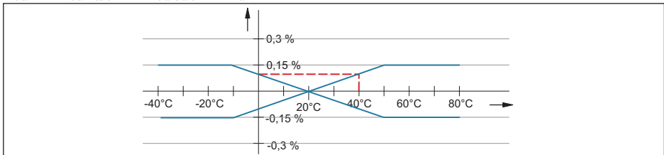
Рис. 26: F_a вследствие термического изменения токового выхода, в этом примере = 0,1 %
