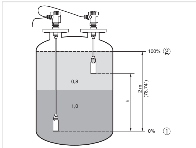
Рис. 21: Пример параметрирования: Установка Min./Max. для измерения межфазного уровня
