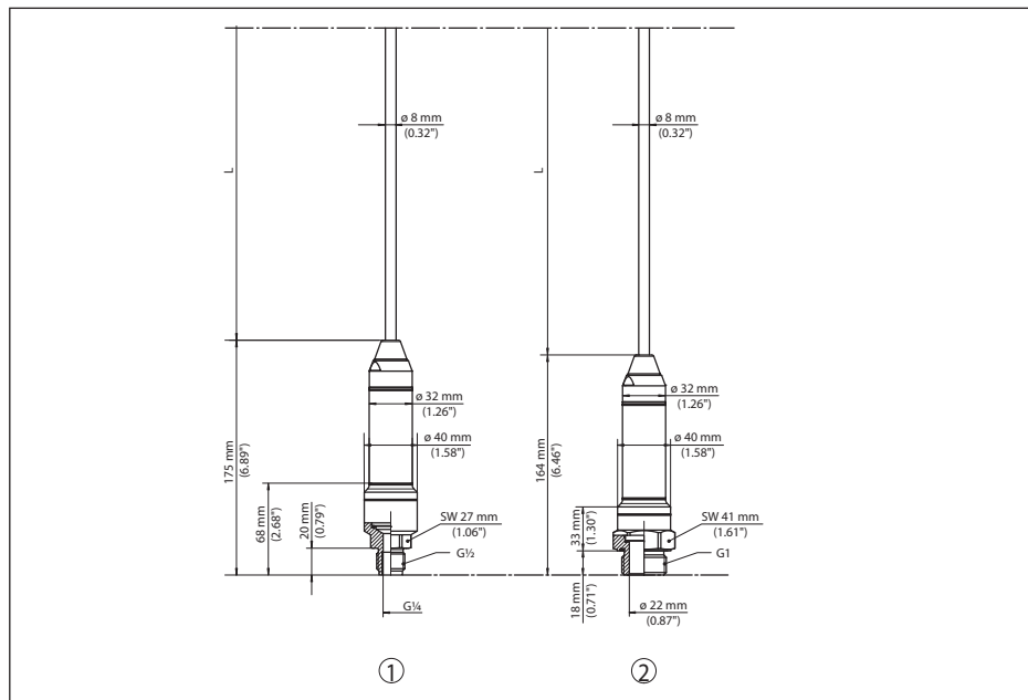
Рис. 34: VEGABAR 86, резьбовое исполнение
