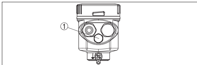
Рис. 8: Положение фильтрующего элемента - исполнение IP 69K 1 Фильтрующий элемент
