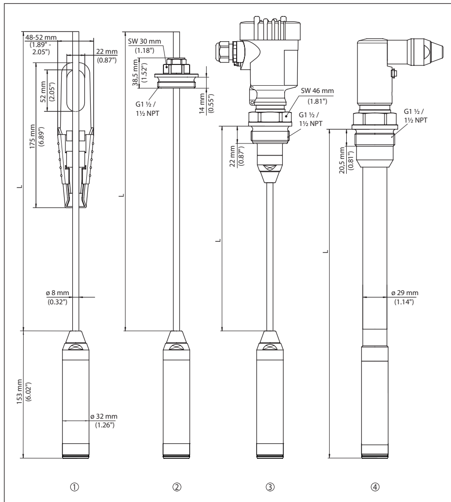
Рис. 30: VEGABAR 86 - чувствительный элемент 32 мм
