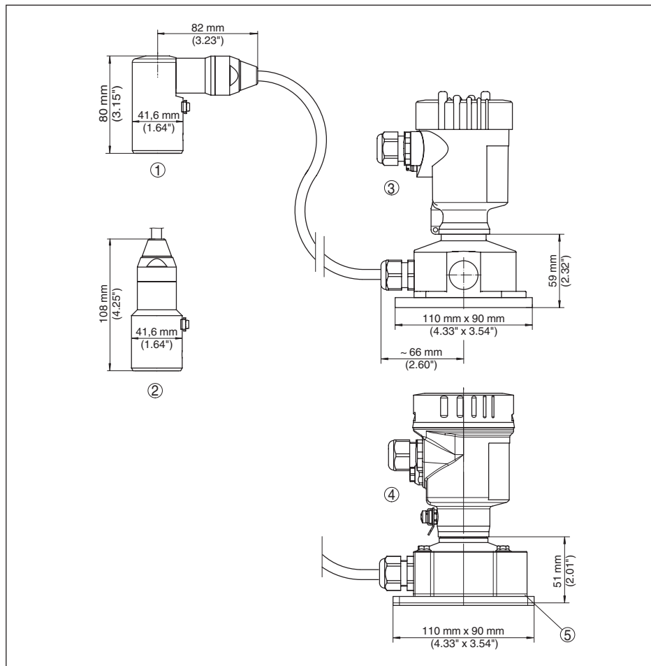
Рис. 28: VEGABAR 86, исполнение IP 68 с выносным корпусом
