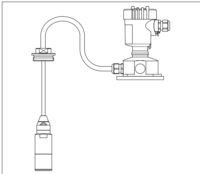
Рис. 16: VEGABAR 86 в исполнении IP 68, 25 bar, без взрывозащиты, с осевым выводом кабеля и выносным корпусом
