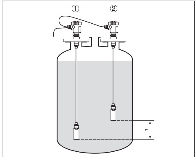
Рис. 12: Измерительная схема для измерения уровня с компенсацией плотности, h = расстояние между двумя точками измерения
