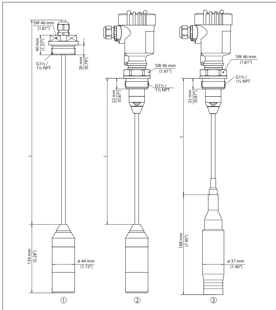
Рис. 31: VEGABAR 86, пластинное исполнение
