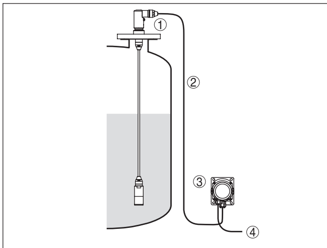
Рис. 13: Схема места измерения, с выносным корпусом
