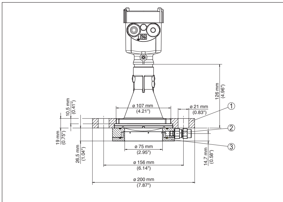
Рис. 79: VEGAPULS 69 с накидным фланцем для фланцев 3" 150 lbs, DN 80 PN 16 м продувочным присоединением
