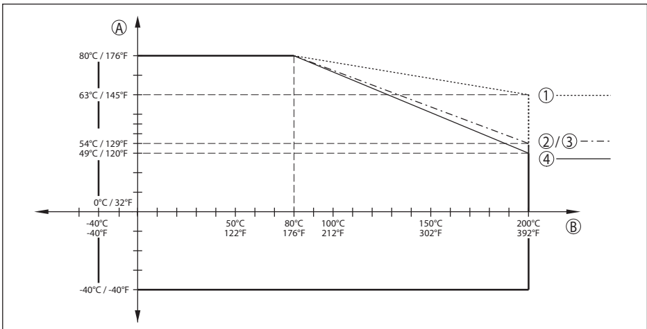
Рис. 56: Снижение номинального значения температуры окружающей среды для исполнения с оправленной металлом линзовой антенной, при температуре процесса до +200 °C (+392 °F)
