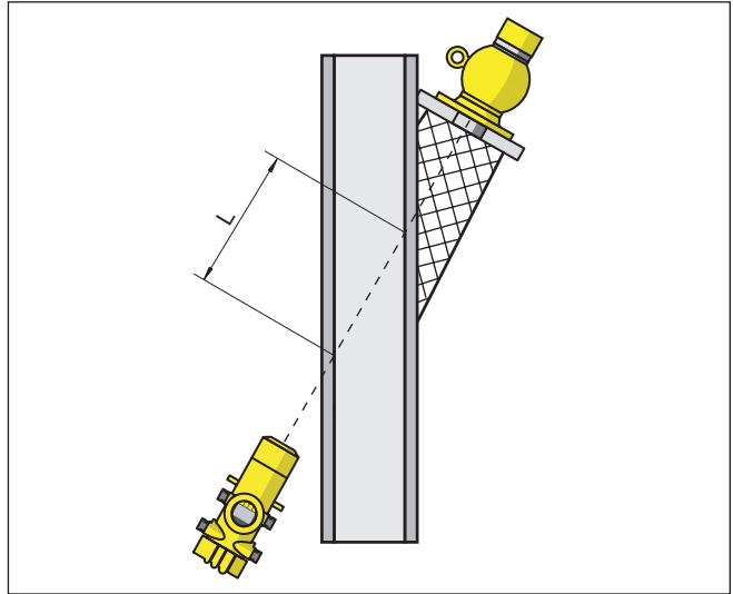
Рис. 22: При косоугольном монтаже применяется длина просвечиваемого отрезка.
