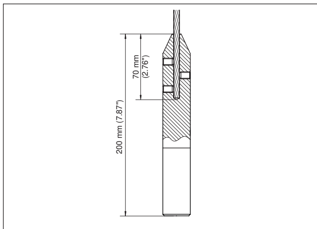
Рис. 20: При укорачивании троса следует учитывать наличие натяжного груза.
