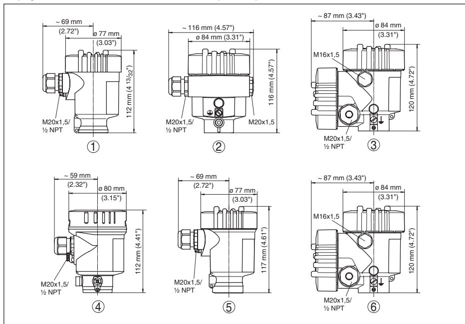
Рис. 27: Корпуса в исполнении IP 66/IP 68 (0,2 bar) - с установленным модулем индикации и настройки корпус выше на 9 мм/0.35 in
