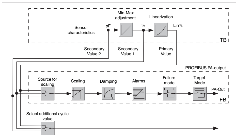
Рис. 22: VEGACAL 67: Блок-схема со значением AI (PA-OUT) и дополнительным циклическим значением
