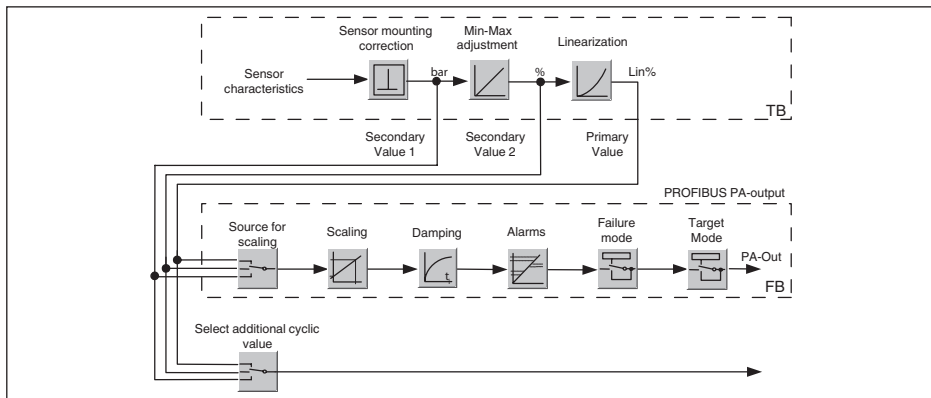
Рис. 57: VEGADIF 65: Блок-схема со значением AI (PA-OUT) и дополнительным циклическим значением (Additional Cyclic Value)
