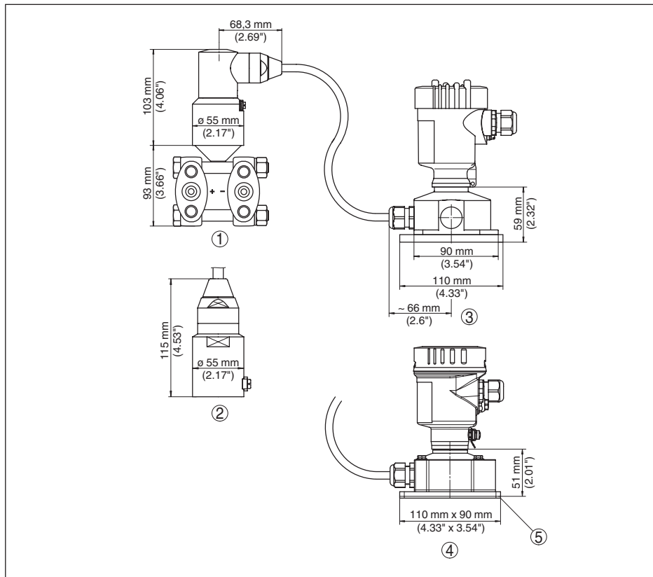
Рис. 68: Выносной корпус
