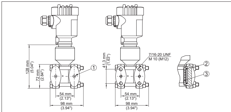
Рис. 71: Слева: Присоединение VEGADIF 65 подготовлено для монтажа изолирующей диафрагмы. Справа: Положение медного уплотнительного кольца
