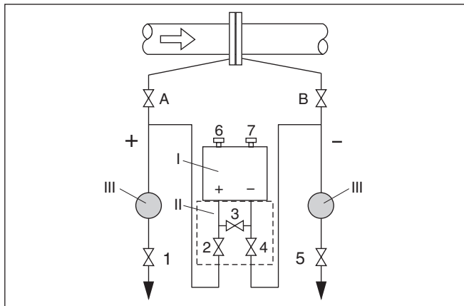
Рис. 52: Предпочтительная схема установки для измерения на жидкостях
