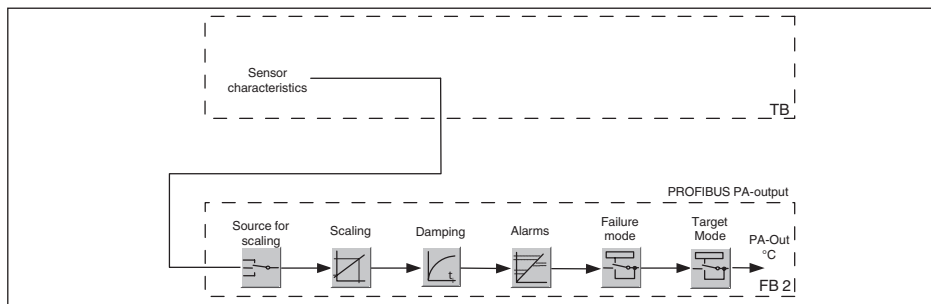
Рис. 58: VEGADIF 65: Блок-схема со значением температуры
