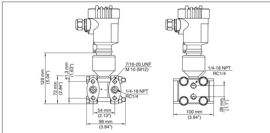
Рис. 70: VEGADIF 65 - присоединение 1/4-18 NPT или RC 1/4, с выпуском воздуха сбоку
