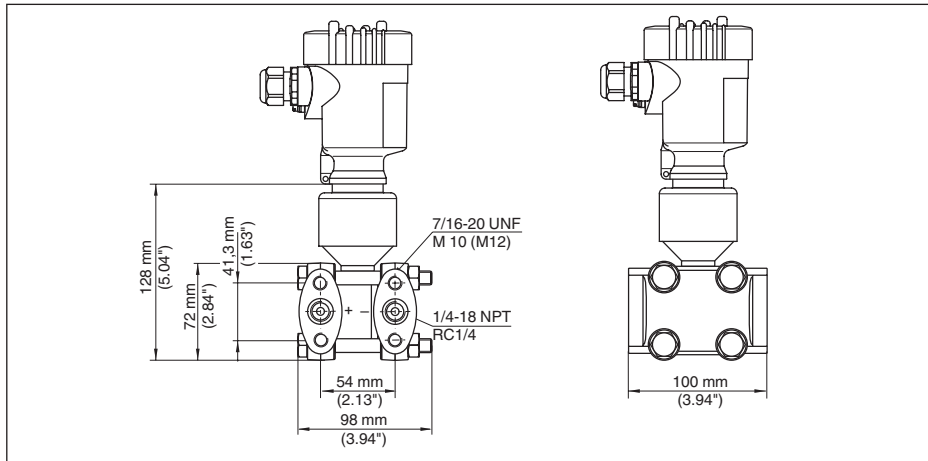
Рис. 69: VEGADIF 65 - присоединение 1/4-18 NPT или RC 1/4
