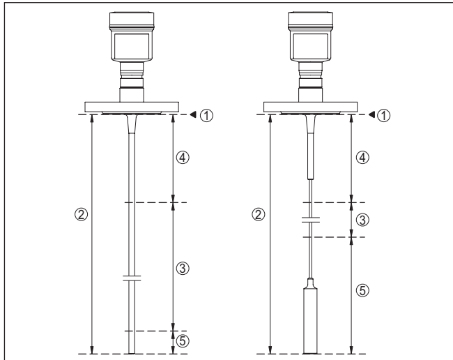
Рис. 12: Диапазоны измерения - VEGAFLEX 83
