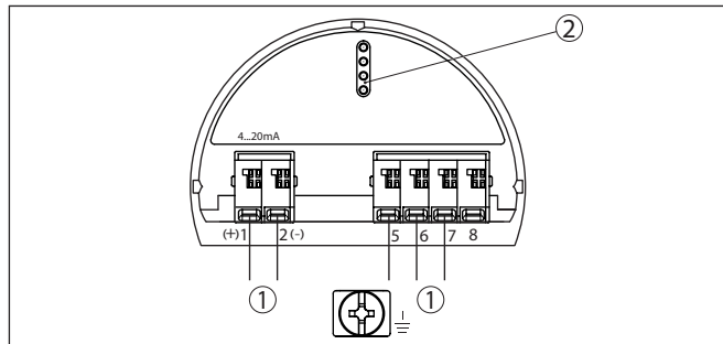
Рис. 4: Отсек электроники (двухкамерный корпус)
