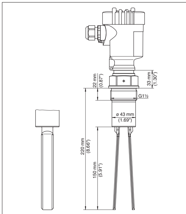
Рис. 52: VEGAWAVE 61, резьбовое исполнение G1 1/2 A (DIN ISO 228/1)
