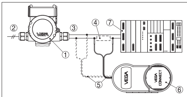
Рис. 19: Подключение ПК к сигнальному кабелю через HART
