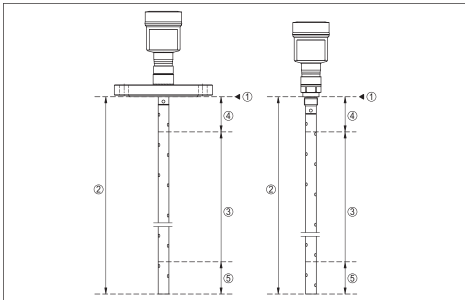
Рис. 32: Диапазоны измерения - VEGAFLEX 81
