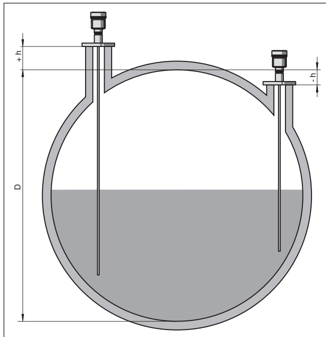
Рис. 17: Высота емкости и значение коррекции патрубка
