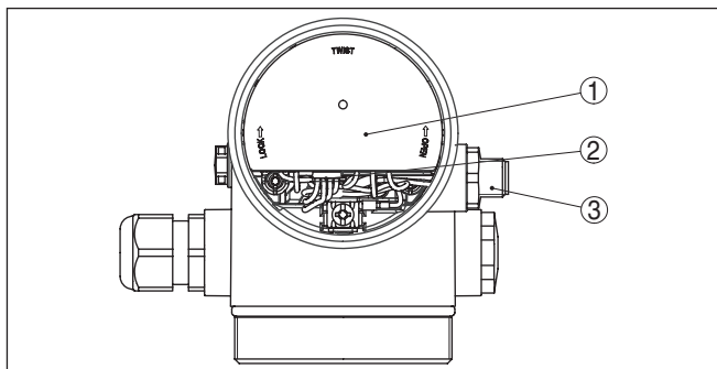
Рис. 11: Вид отсека электроники с адаптером VEGADIS для подключения выносного устройства индикации и настройки
