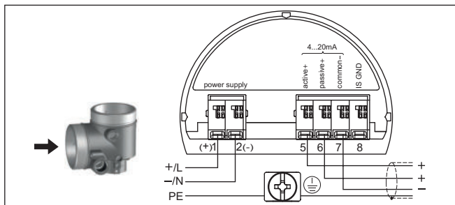
Рис. 9: Отсек подключения в двухкамерном корпусе в случае сетевого напряжения
