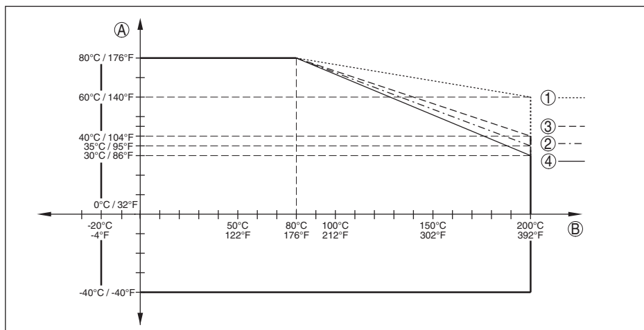
Рис. 36: Температура окружающей среды - температура процесса, исполнение с температурной вставкой
