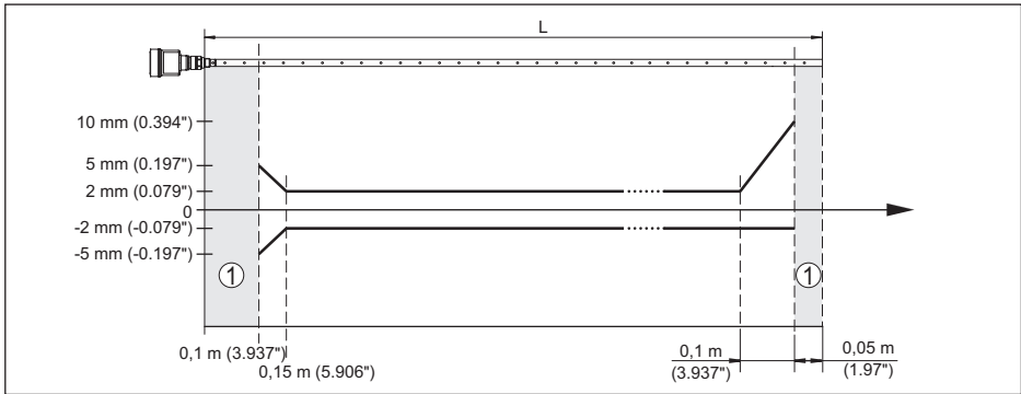
Рис. 34: Погрешность измерения VEGAFLEX 81 в коаксиальном исполнении (среда - масло)
