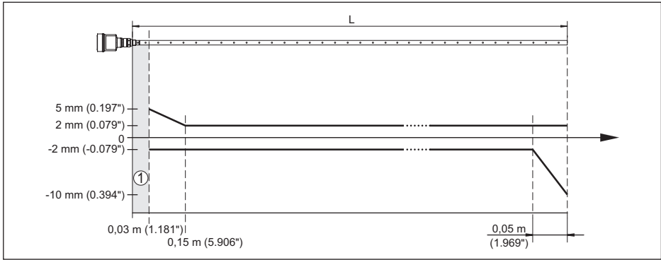
Рис. 33: Погрешность измерения VEGAFLEX 81 в коаксиальном исполнении (среда - вода)
