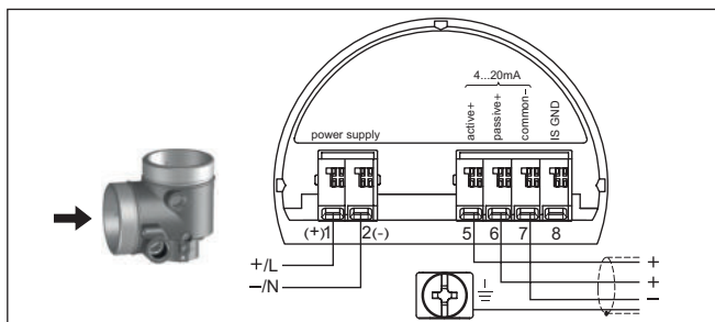
Рис. 10: Отсек подключения в двухкамерном корпусе в случае малого напряжения
