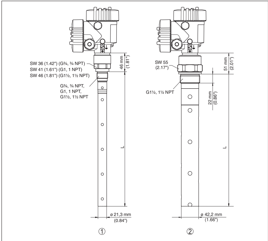
Рис. 38: VEGAFLEX 81, резьбовое исполнение
