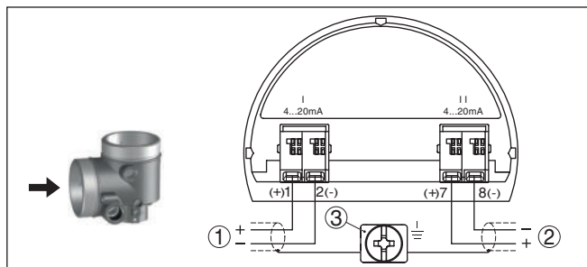
Рис. 13: Отсек подключения в двухкамерном корпусе, дополнительная электроника "Дополнительный токовый выход"
