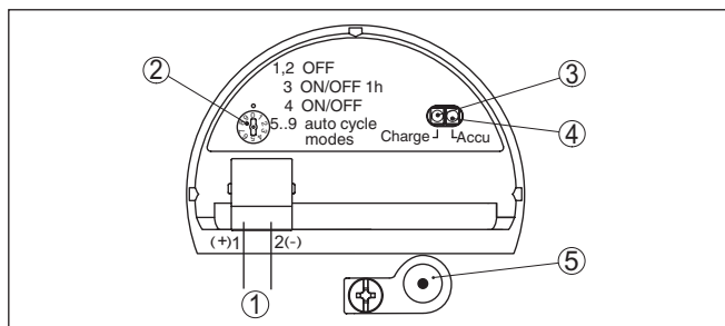
Рис. 3: Отсек питания
