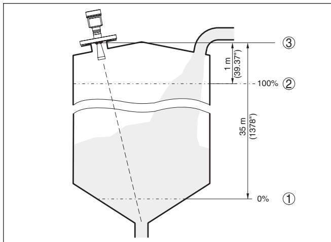
Рис. 11: Пример параметрирования
