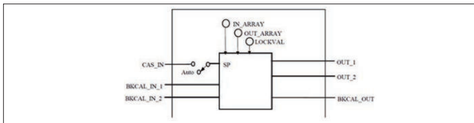
Рис. 55: Схема функционального блока Output Splitter
