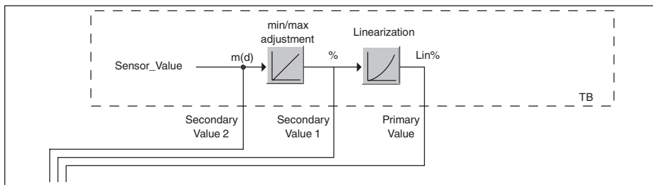
Рис. 51: Схематическое представление блока преобразователя (TB)
