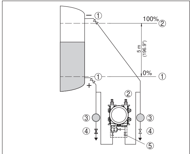
Рис. 41: Пример параметрирования: Установка Min./Max. для измерения уровня
