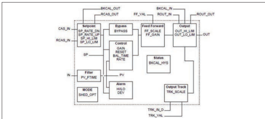
Рис. 54: Схема функционального блока PID Control
