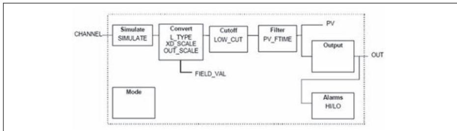
Рис. 52: Схема функционального блока Analog Input (AI)
