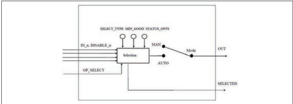
Рис. 58: Схема функционального блока Input Selector
