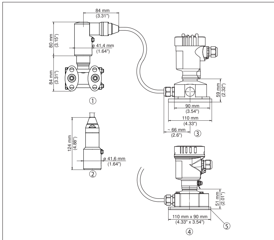
Рис. 64: Выносной корпус
