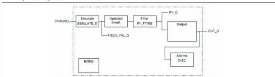
Рис. 53: Схема функционального блока Discret Input (DI)
