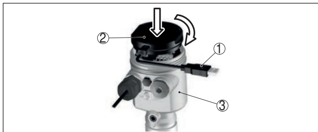
Рис. 42: Подключение ПК через интерфейсный адаптер прямо к датчику
