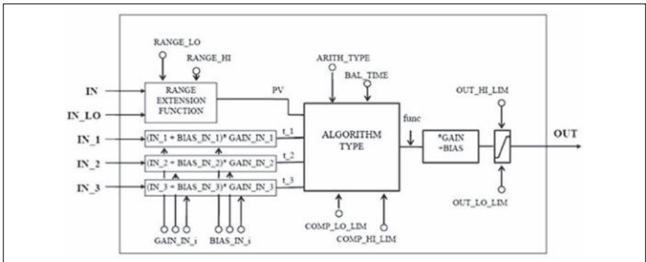
Рис. 59: Схема функционального блока Arithmetic
