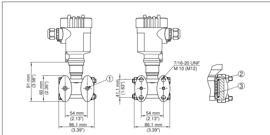
Рис. 67: Слева: Присоединение VEGADIF 85 подготовлено для монтажа изолирующей диафрагмы. Справа: Положение медного уплотнительного кольца
