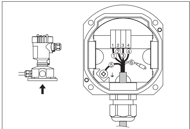
Рис. 35: Подключение рабочего узла в цоколе корпуса
