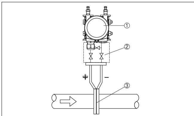
Рис. 17: Схема установки для измерения расхода на газax, подключение через 3-вентильный блок с фланцевым присоединением с обеих сторон
