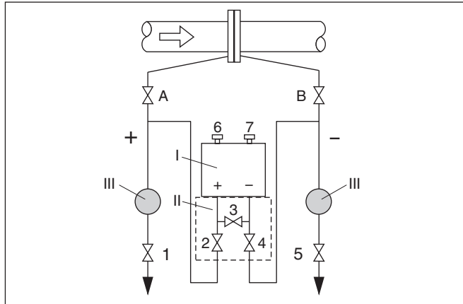
Рис. 47: Предпочтительная схема установки для измерения на жидкостях
