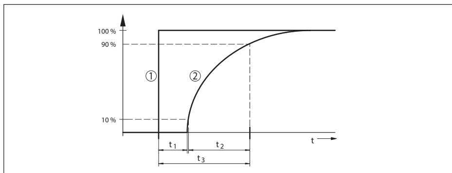
Рис. 50: Состояние при скачкообразном изменении параметров процесса. t_1 : время нечувствительности; t_2 : время нарастания; t_3 : время реакции на скачкообразное изменение
