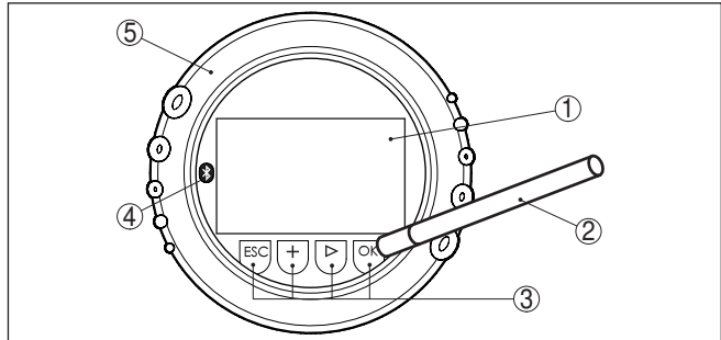
Рис. 40: Элементы индикации и настройки - настройка посредством магнитного карандаша
