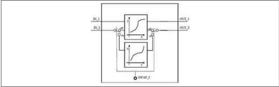
Рис. 56: Схема функционального блока Signal Characterizer
