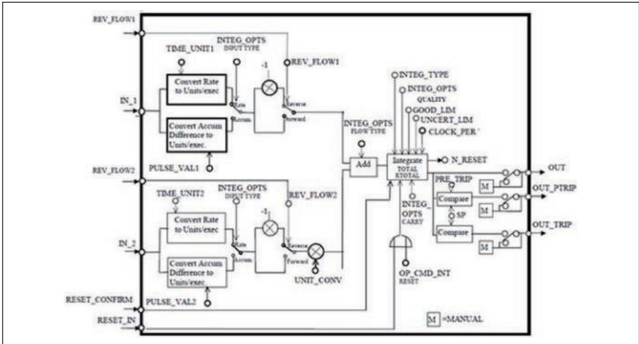
Рис. 57: Схема функционального блока Integrator
