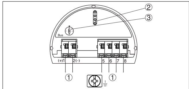
Рис. 31: Отсек электроники (двухкамерный корпус)
