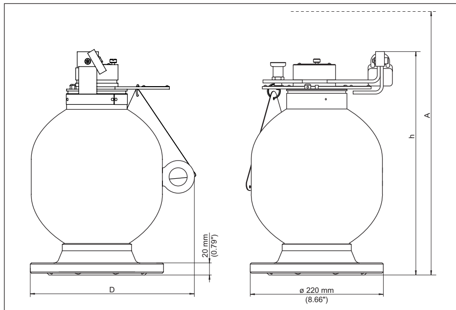
Рис. 41: Держатель источника VEGASOURCE 35 - Исполнение В (поворотный бугель для ручного переключения ВКЛ/ВЫКЛ, фиксатор для заперения положения ВКЛ, висячий замок для заперения положения ВЫКЛ)
