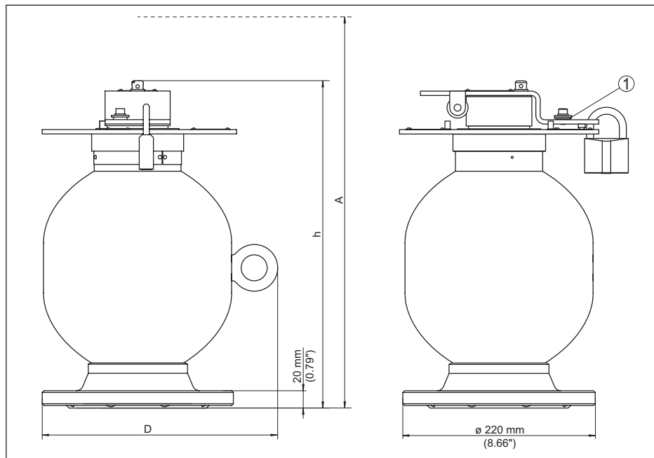
Рис. 43: Держатель источника VEGASOURCE 35 - Исполнение D
