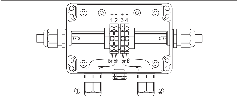
Рис. 24: Соединительная клеммная коробка бесконтактных переключателей
