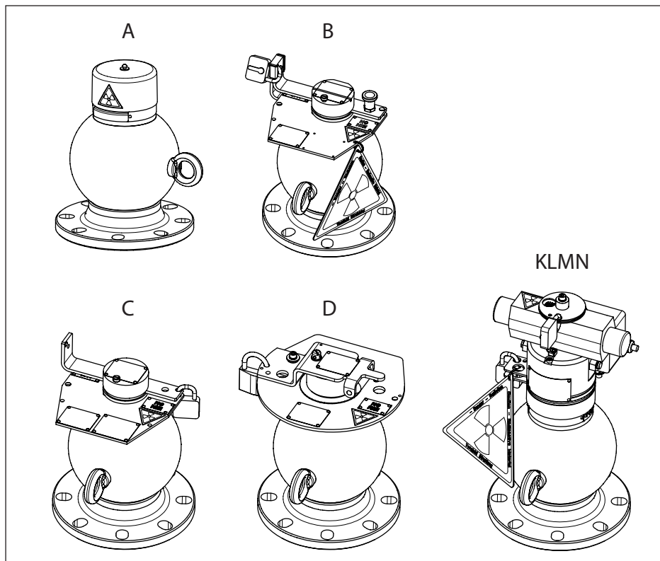
Рис. 2: Исполнения VEGASOURCE 35 - общий обзор
