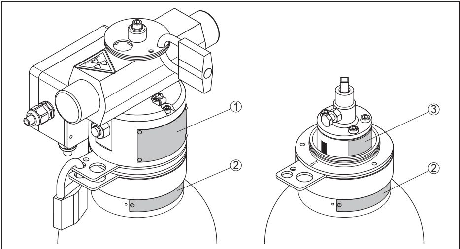
Рис. 7: Положение типовых шильдиков - Исполнения К L M N
