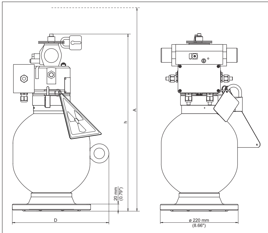
Рис. 44: Держатель источника VEGASOURCE 35 - Исполнение К и L
