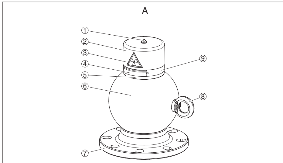
Рис. 33: Материалы VEGASOURCE 35 - Исполнение устройства А
