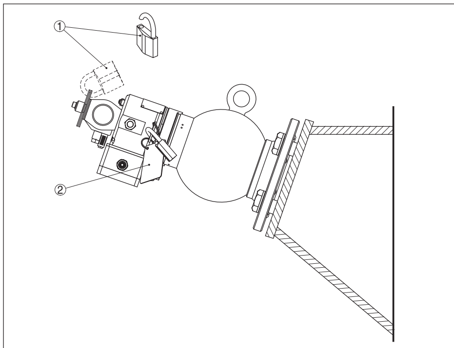
Рис. 30: Включение излучения посредством пневматического устройства - VEGASOURCE 35 в исполнении К, L, М, N
