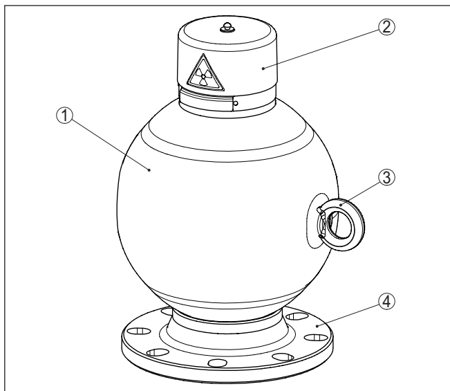
Рис. 9: Защитный держатель источника VEGASOURCE 35
