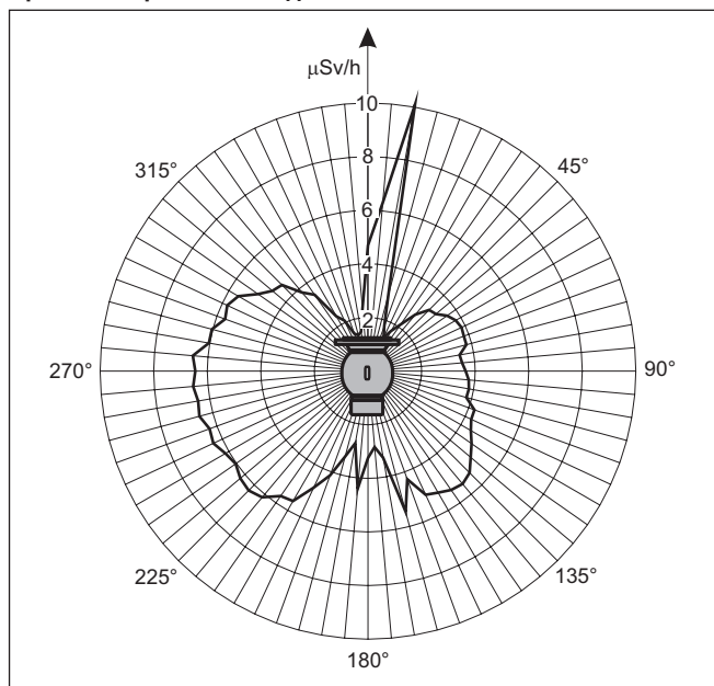
Рис. 38: Кривая изорасстояния (расстояние: 1 м) - пример: держатель источника VEGASOURCE 35 с Co-60, 100 мКи (3,7 ГБк)
