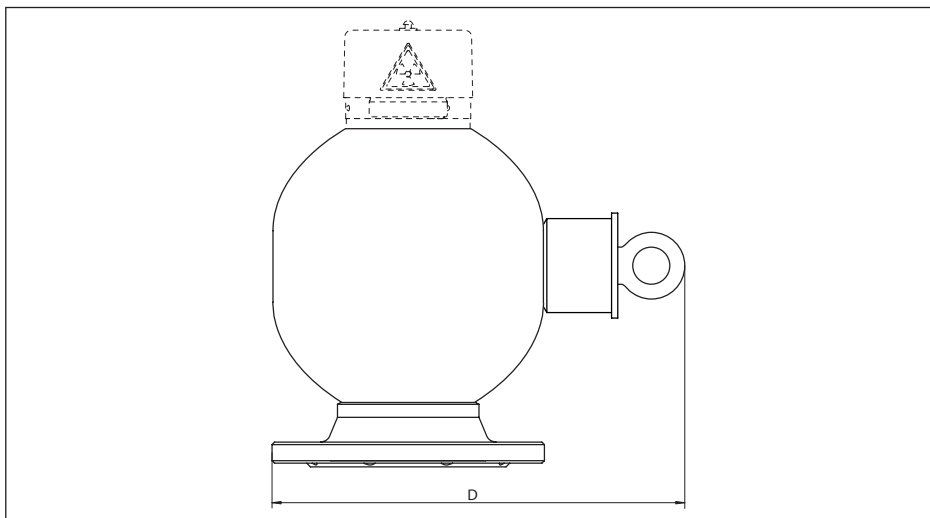
Рис. 47: Держатель источника VEGASOURCE 35 - огнестойкое исполнение (вариант)
