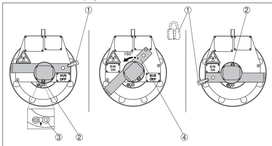
Рис. 28: Включение излучения - VEGASOURCE 35 Исполнение С
