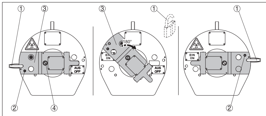
Рис. 29: Включение излучения - VEGASOURCE 35 Исполнение D
