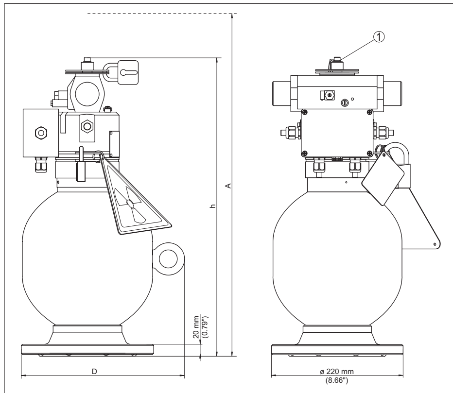
Рис. 45: Держатель источника VEGASOURCE 35 - Исполнение М и N
