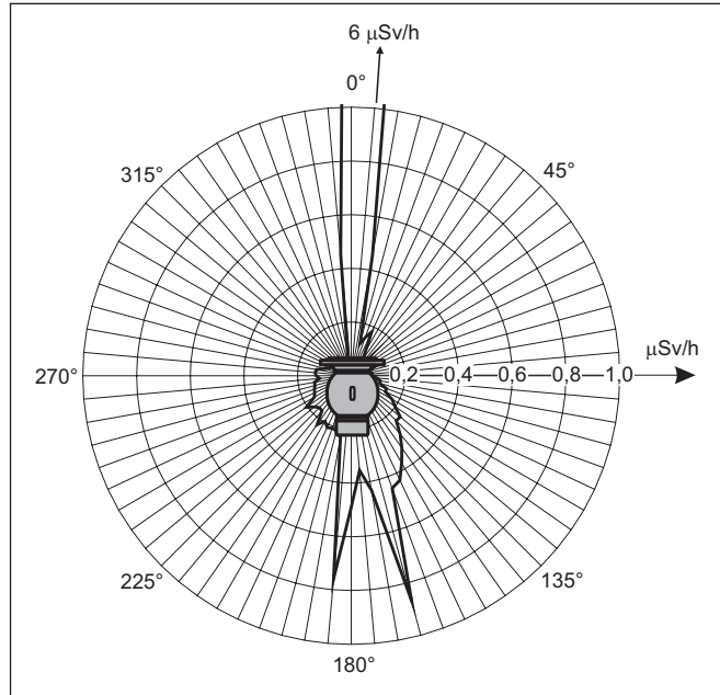
Рис. 39: Кривая изорасстояния (расстояние: 1 м) - пример: держатель источника VEGASOURCE 35 с Cs-137, 1000 мКи (37 ГБк)
