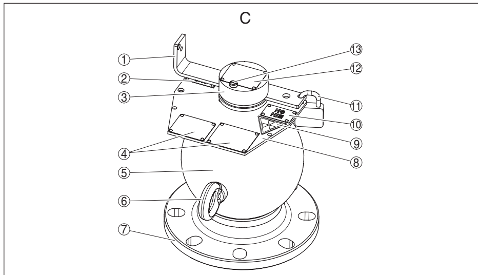
Рис. 35: Материалы VEGASOURCE 35 - Исполнение устройства С
