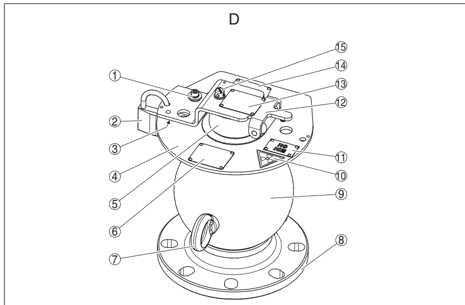
Рис. 36: Материалы VEGASOURCE 35 - Исполнение устройства D
