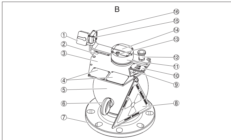
Рис. 34: Материалы VEGASOURCE 35 - Исполнение устройства В
