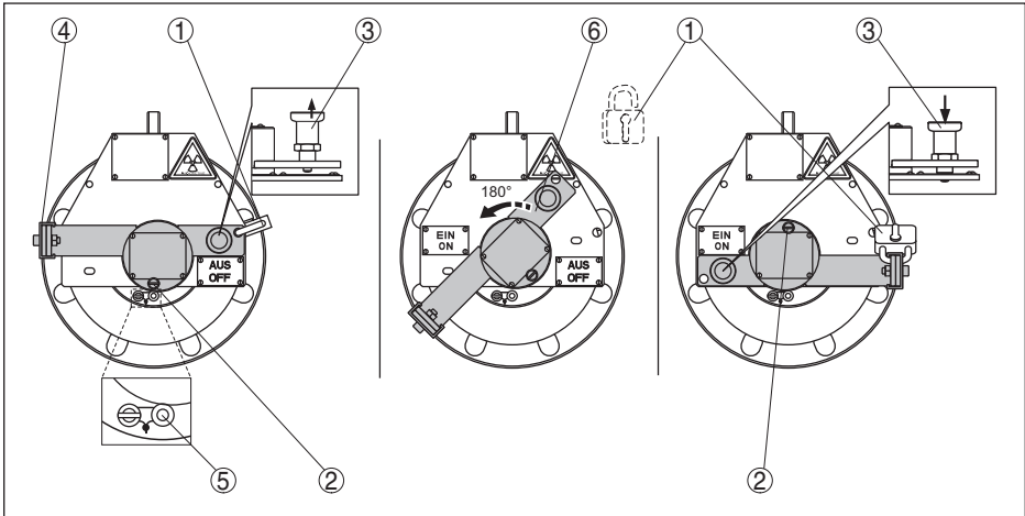
Рис. 27: Включение излучения - VEGASOURCE 35 Исполнение В
