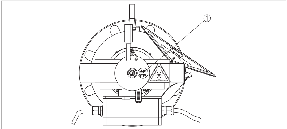
Рис. 31: Индикация состояния переключения у VEGASOURCE 35 в исполнении K, L, M, N
