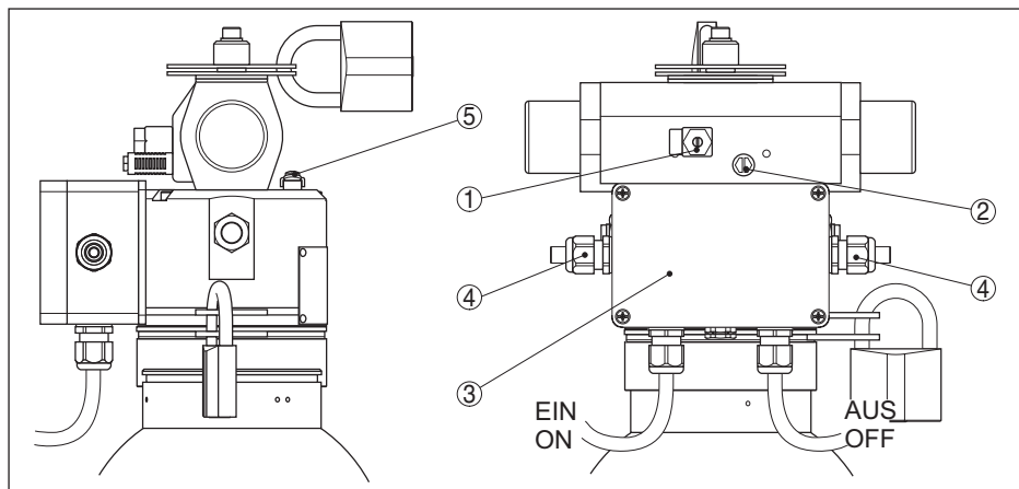
Рис. 25: Подключение пневмолиний к VEGASOURCE 35 - исполнения K L M N
