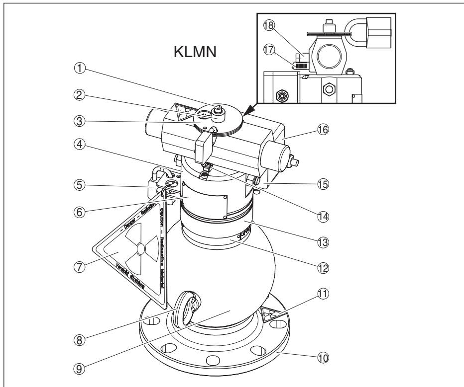
Рис. 37: Материалы VEGASOURCE 35 - Исполнение K L M N
