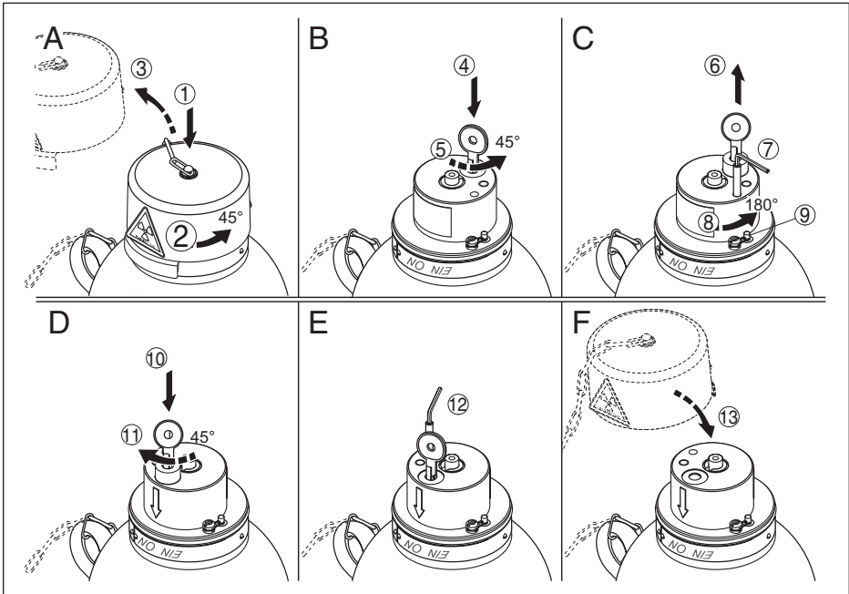
Рис. 26: Включение излучения - VEGASOURCE 35 Исполнение А
