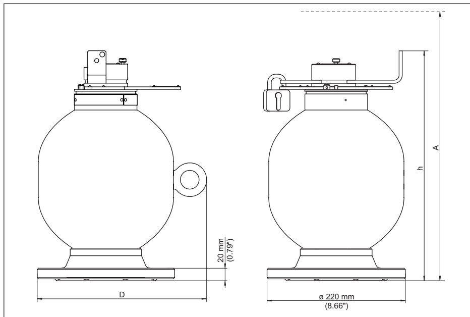
Рис. 42: Держатель источника VEGASOURCE 35 - Исполнение С (поворотный бугель для ручного переключения ВКЛ/ВЫКЛ, висячий замок для заперения положения ВЫКЛ или ВЫКЛ)
