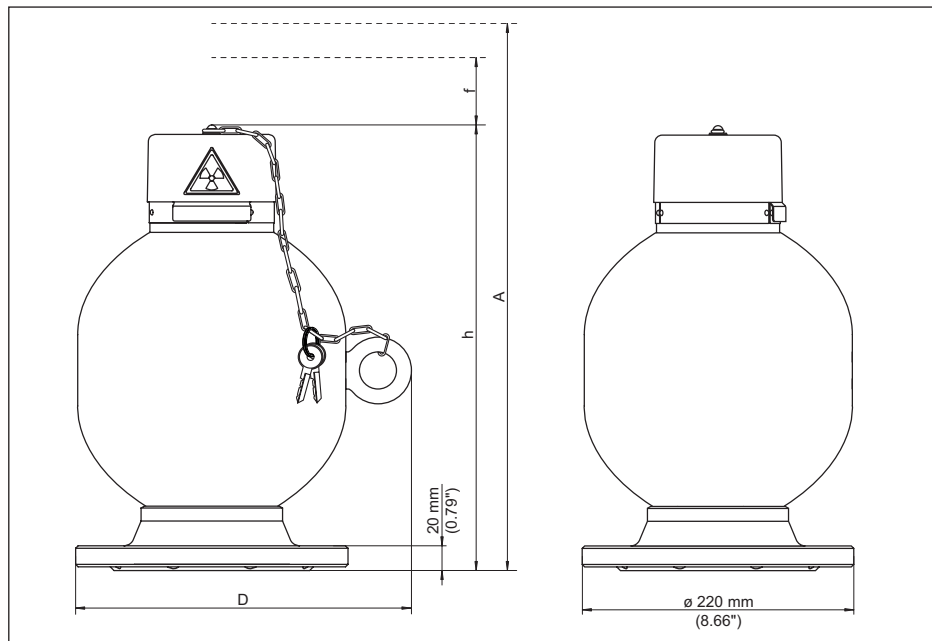
Рис. 40: Держатель источника VEGASOURCE 35 - Исполнение А (вставка с препаратом с ручным переключением ВКЛ/ВЫКЛ, вставной замок для запираения положения ВКЛ или ВЫКЛ, защитный кожух)
