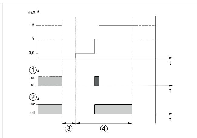
Рис. 6: Диаграмма ошибочного импульса включения
