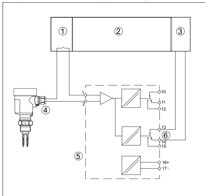
Рис. 4: Автоматизированная функциональная проверка через реле сигнала неисправности и ПЛК
