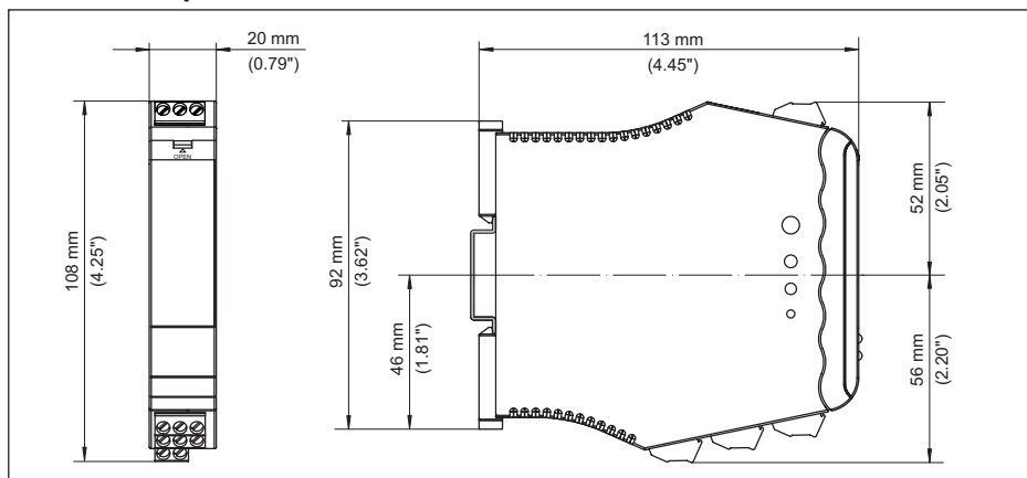
Рис. 23: Размеры VEGATOR 121
