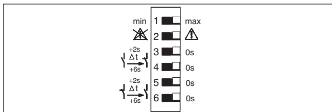
Рис. 3: DIL-переключатель VEGATOR 121
