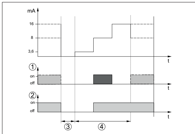
Рис. 5: Диаграмма правильного импульса включения
