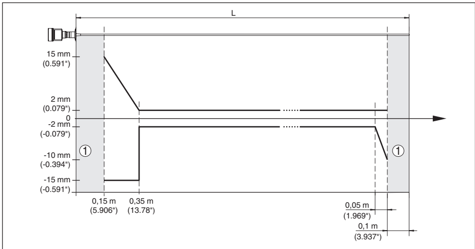
Рис. 44: Погрешность измерения VEGAFLEX 83 в стержневом исполнении (среда - масло)
