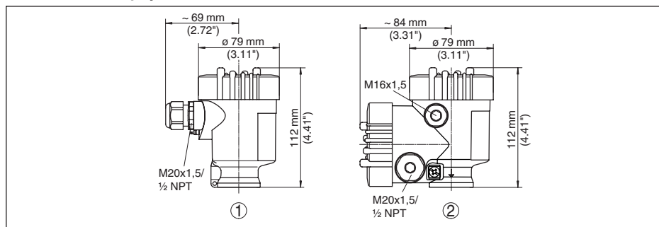
Рис. 46: Корпуса в исполнении со степенью защиты IP 66/IP 67 (с установленным модулем индикации и настройки корпус выше на 9 мм/0.35 in)
