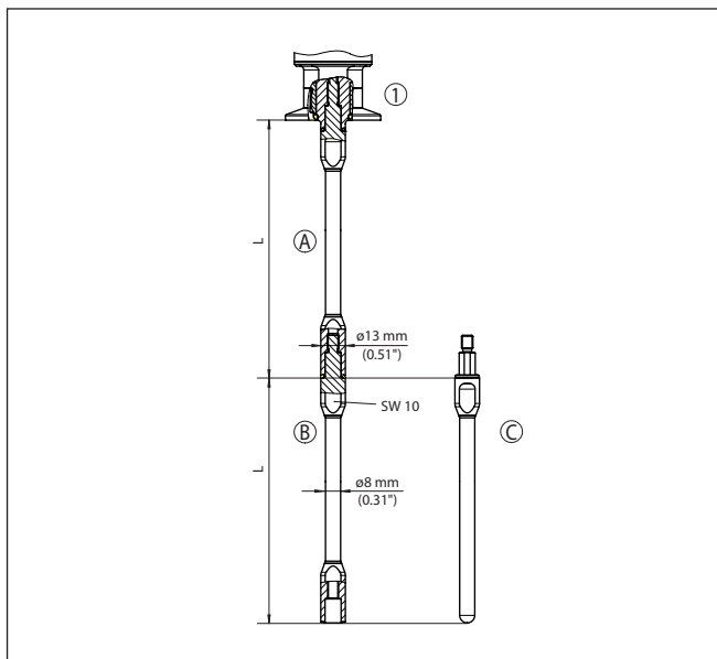
Рис. 53: Удлинительные сегменты стержня \varnothing 8 мм (0.315 in)
