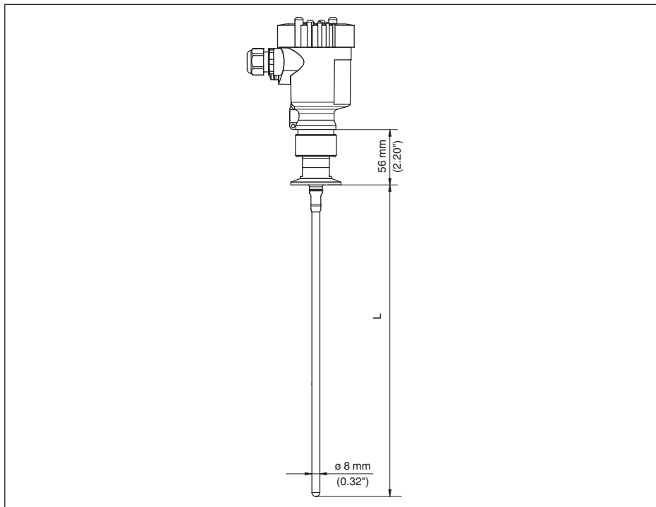
Рис. 51: VEGAFLEX 83, стержневое исполнение \varnothing 8 mm (0.315 in), полированный
