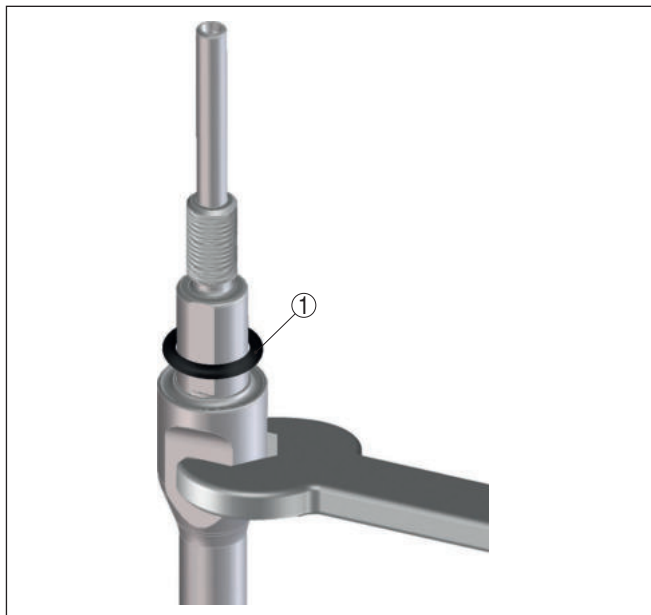
Рис. 39: Замена измерительного стержня
