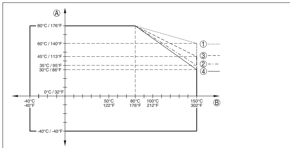
Рис. 45: Температура окружающей среды - температура процесса, стандартное исполнение
