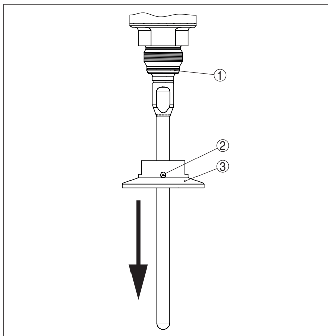
Рис. 41: Уплотнение присоединения к процессу
