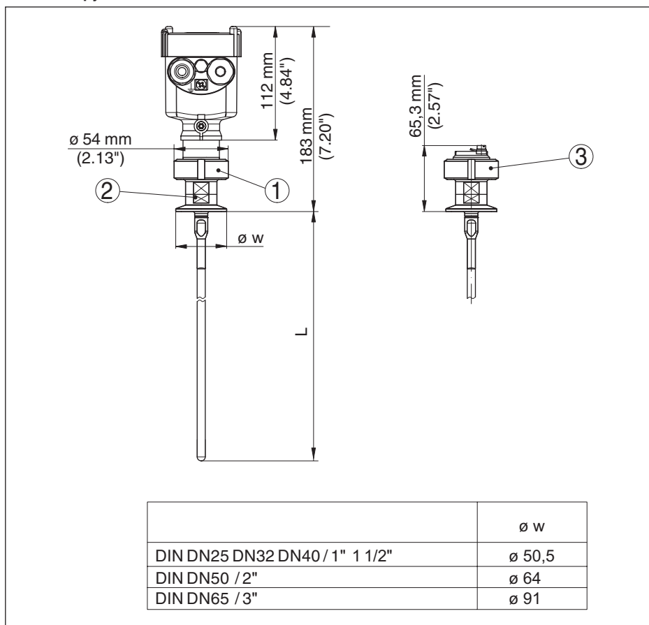
Рис. 52: VEGAFLEX 83, стержневое исполнение \varnothing 8 mm (0.315 in), полированное - автоклавируемое исполнение
