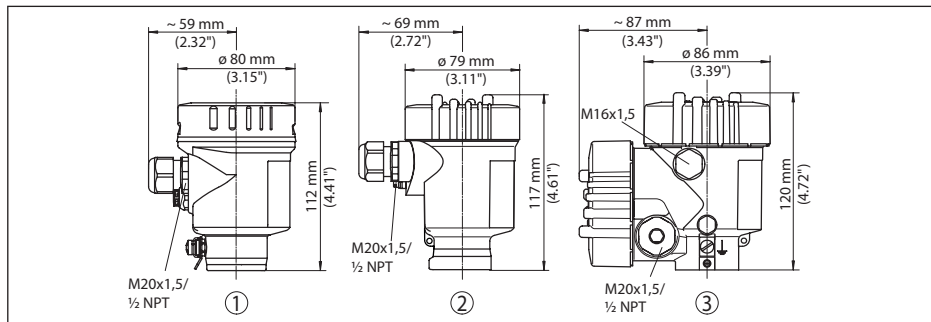
Рис. 49: Корпуса в исполнении IP 66/IP 68 (0,2 bar) - с установленным модулем индикации и настройки корпус выше на 9 мм/0.35 in
