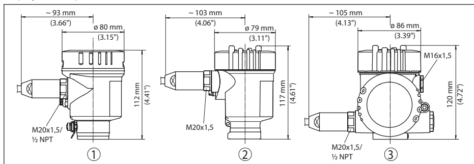
Рис. 50: Корпуса в исполнении IP 66/IP 68 (1 bar) - с установленным модулем индикации и настройки корпус выше на 9 мм/0.35 in
