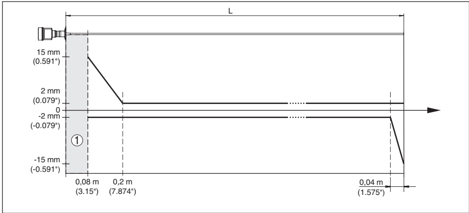
Рис. 43: Погрешность измерения VEGAFLEX 83 в стержневом исполнении (среда - вода)
