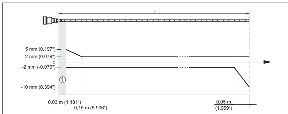
Рис. 34: Погрешность измерения VEGAFLEX 81 в коаксиальном исполнении (среда - вода)
