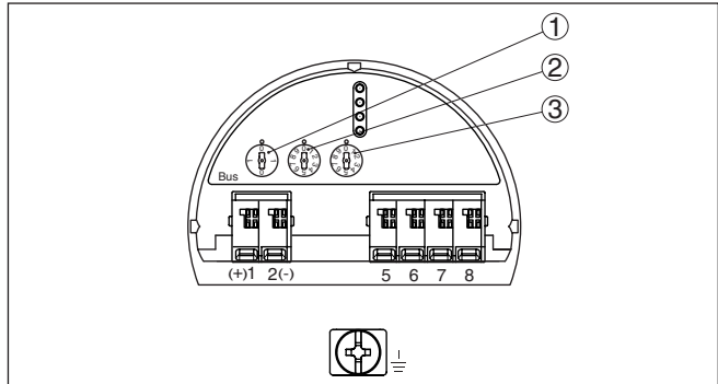
Рис. 15: Переключатели выбора адреса
