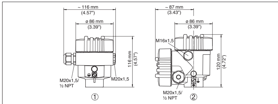
Рис. 42: Корпуса в исполнении IP 66/IP 68 (0,2 bar) - с установленным модулем индикации и настройки корпус выше на 9 mm/0.35 in
