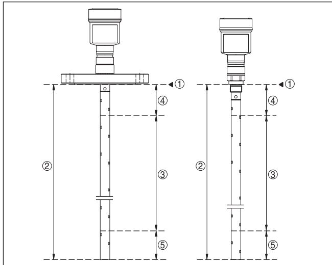
Рис. 9: Диапазоны измерения - VEGAFLEX 81
