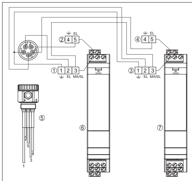
Рис. 2: Схема подключения VEGATOR 132
