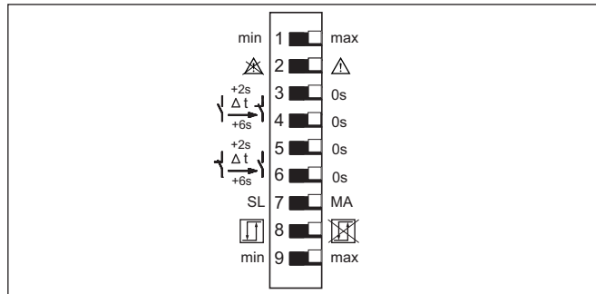
Рис. 4: DIL-переключатель VEGATOR 132
