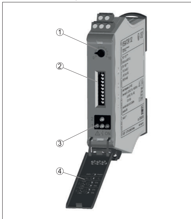
Рис. 3: Элементы индикации и настройки
