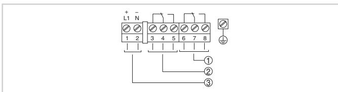
Схема подключения
