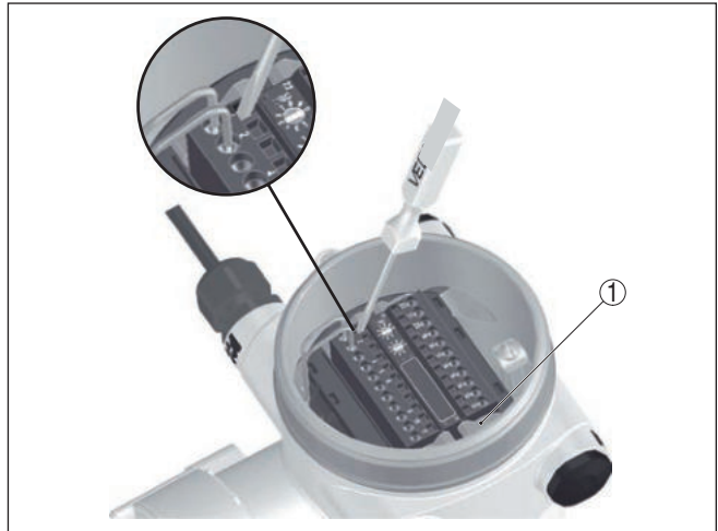
Рис. 7: Подключение: шаги 4 и 5
