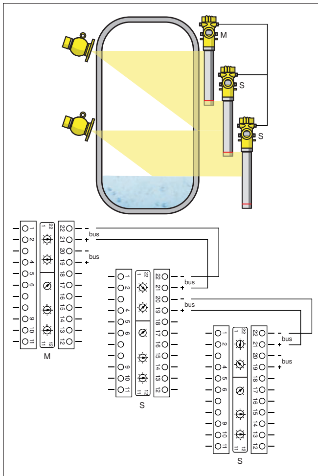
Рис. 16: Отсек электроники и подключения при каскадной установке нескольких устройств
