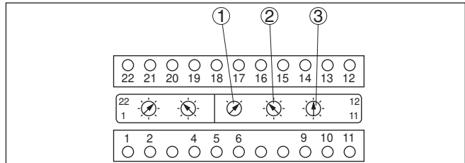
Рис. 17: Переключатели выбора адреса
