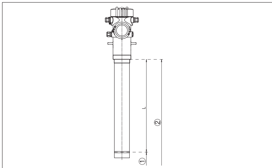
Рис. 24: Данные для входной величины
