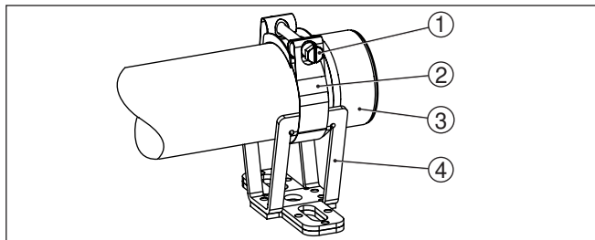
Рис. 4: Монтажный хомут
