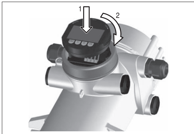
Рис. 18: Установка модуля индикации и настройки
