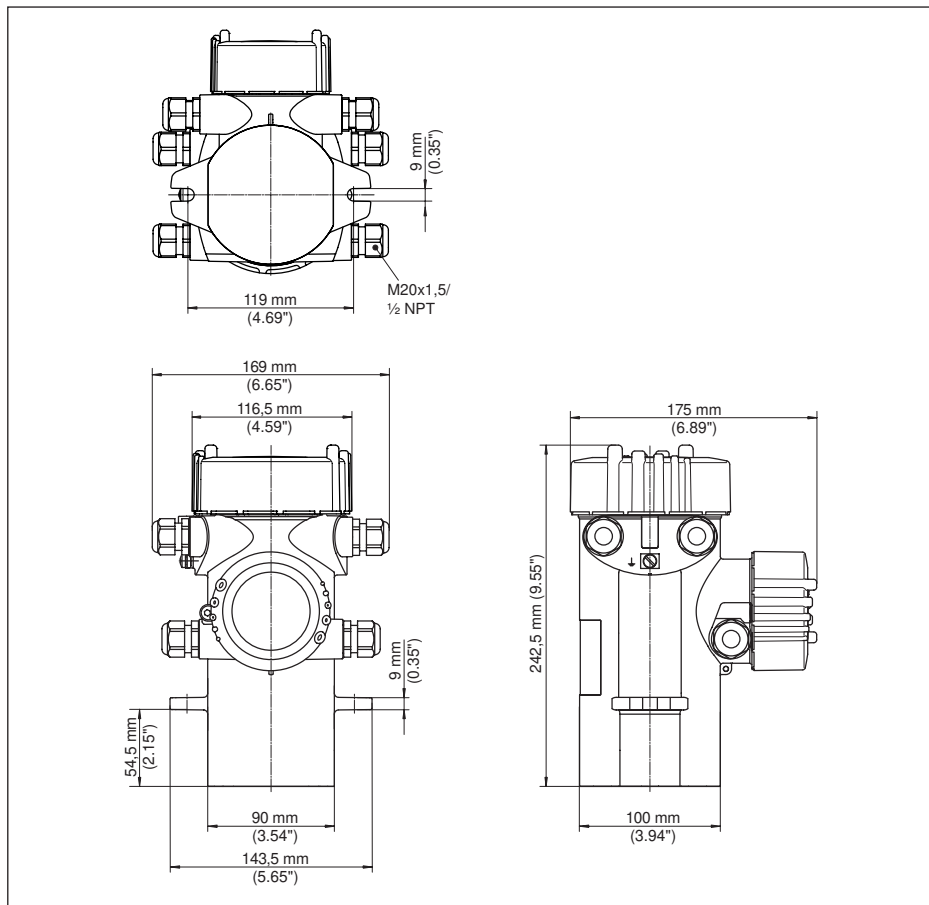
Рис. 32: Корпус из алюминия или нержавеющей стали (точное литье)
