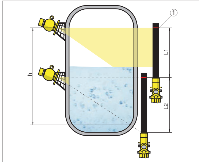
Рис. 5: Монтажное положение - каскадная установка
