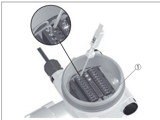
Рис. 7: Подключение: шаги 4 и 5
