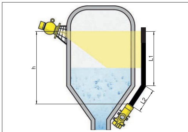
Рис. 3: Измерение уровня в резервуаре-хранилище
