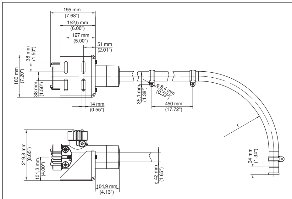
Рис. 34: FIBERTRAC 31 с поставляемыми в комплекте монтажными принадлежностями
