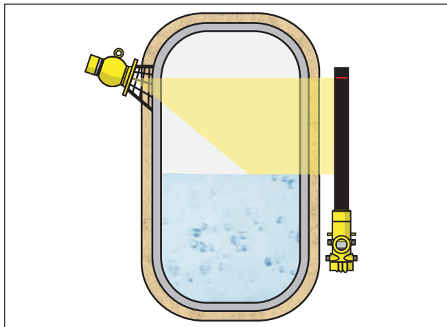
Рис. 6: Измерение уровня в обогреваемой емкости с теплоизоляцией
