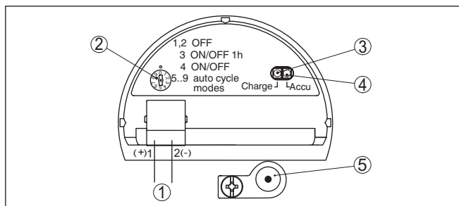
Рис. 6: Отсек питания
