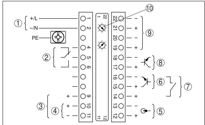
Рис. 10: Отсек электроники и подключения у устройств без взрывозащиты и устройств с не искробезопасным токовым выходом
