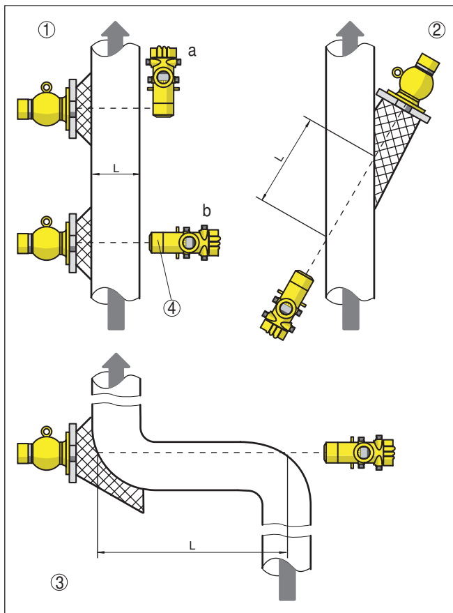
Рис. 5: Варианты монтажа для измерения плотности или концентрации 1a Радиальное просвечивание - вертикальный монтаж 1b Осевое просвечивание - горизонтальный монтаж или при применении свинцового кожуха для защиты от фонового излучения 2 Косоугольное просвечивание для увеличения просвечиваемой длины (L) 3 Увеличение просвечиваемой длины (L) посредством вставки колена трубопровода как измерительного отрезка 4 Встроенный свинцовый кожух для защиты от фонового излучения - прибор экранирован сбоку
