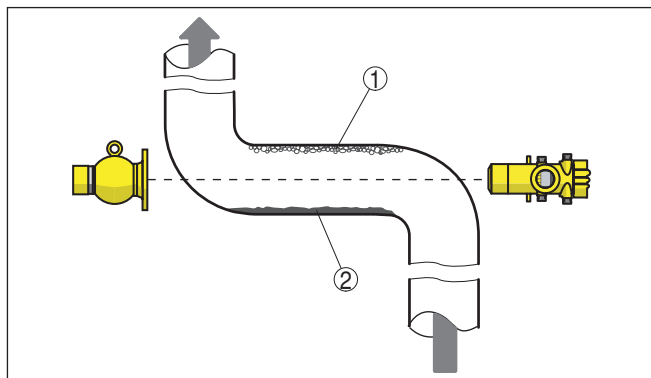
Рис. 4: Монтаж на горизонтальном трубопроводе
