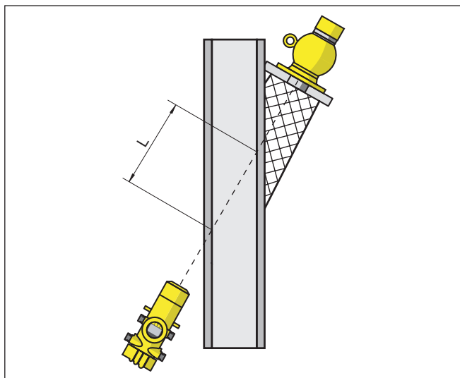
Рис. 21: При косоугольном монтаже применяется длина просвечиваемого отрезка.
