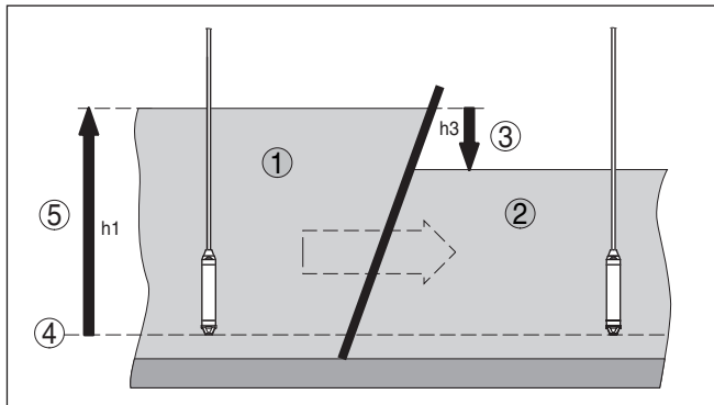
Рис. 12: Измерение разности для управления плотиной
