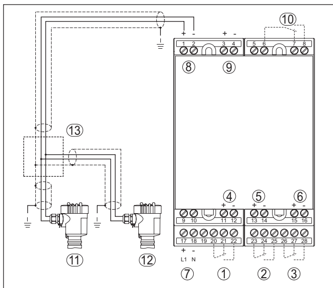
Рис. 3: Схема подключения VEGAMET 625 с двухпроводными датчиками
