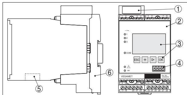
Рис. 1: VEGAMET 625
