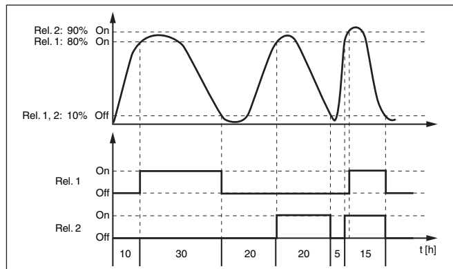
Рис. 14: Пример управления насосами 2
