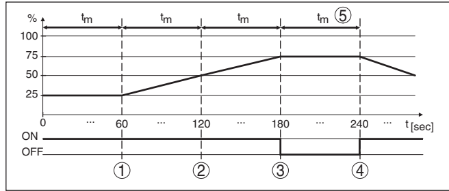
Рис. 15: Пример сигнализации тенденции
