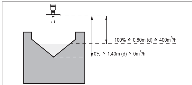
Рис. 16: Установка для измерения расхода с треугольным водосливом
