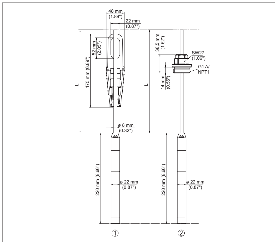
Рис. 16: VEGAWELL 52, с чувствительным элементом из 316L/титана, 22 мм
