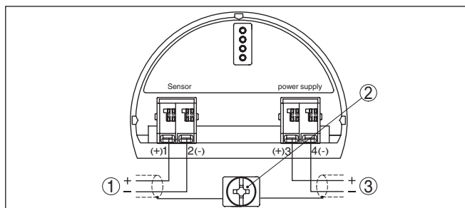
Рис. 13: Схема подключения VEGAWELL 52 для датчиков 4 ... 20 mA
