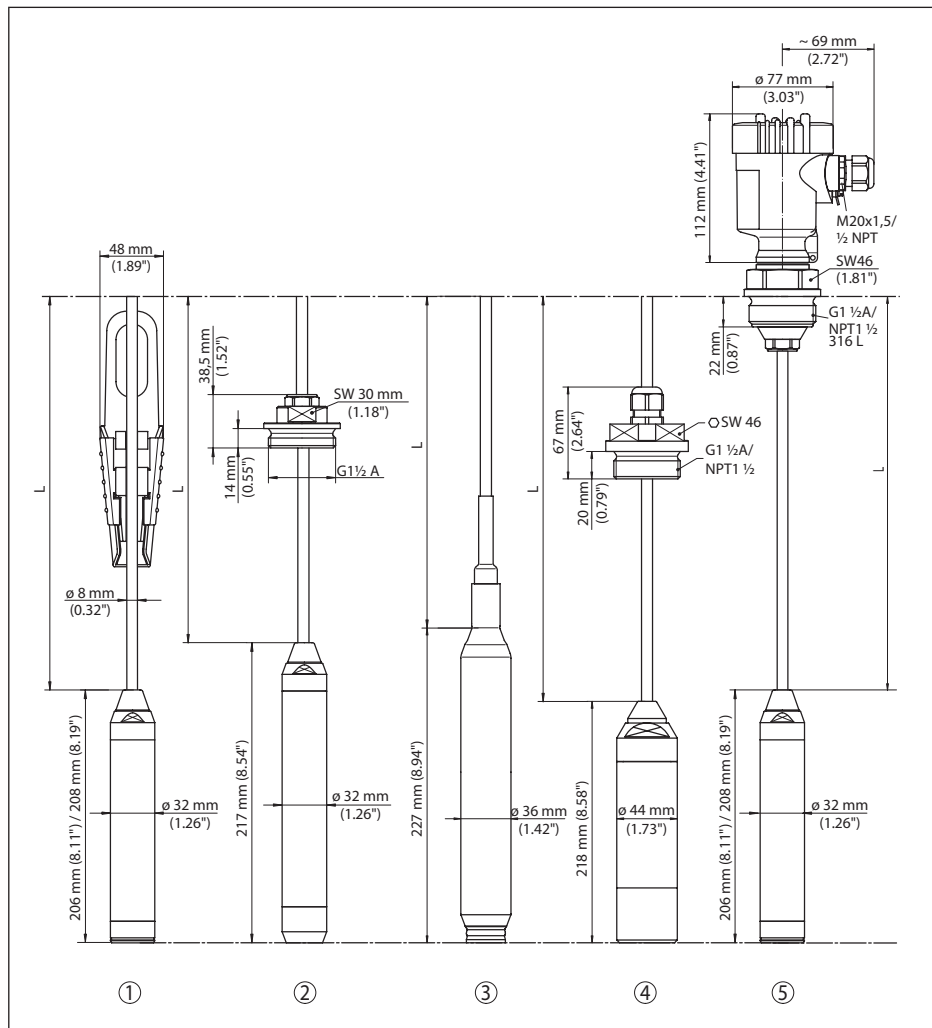
Рис. 18: VEGAWELL 52, с чувствительным элементом из дуплексной стали (1.4462)/PVDF
