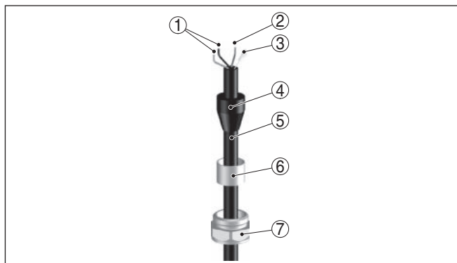
Рис. 15: Структура уплотнения кабеля
