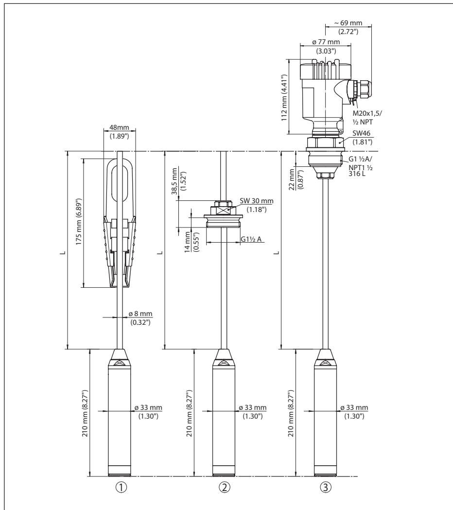
Рис. 17: VEGAWELL 52, с чувствительным элементом из титана, 33 мм
