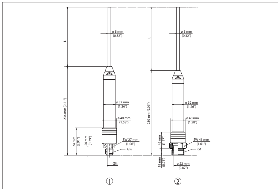
Рис. 19: VEGAWELL 52, с резьбовым присоединением и чувствительным элементом из дуплексной стали (1.4462)
