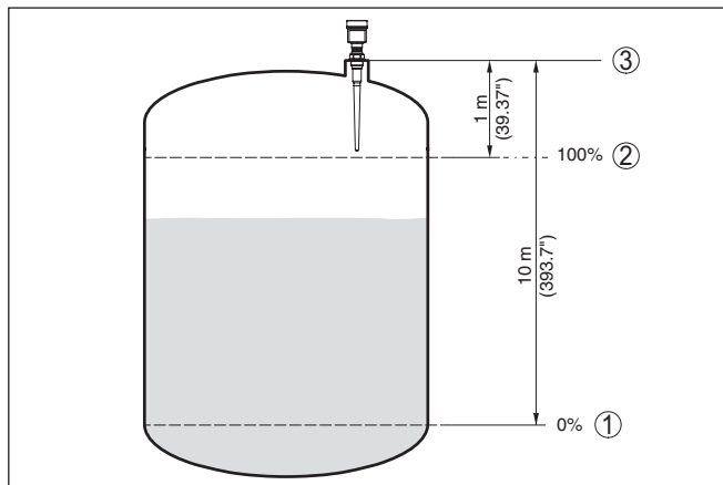
Рис. 7: Пример параметрирования
