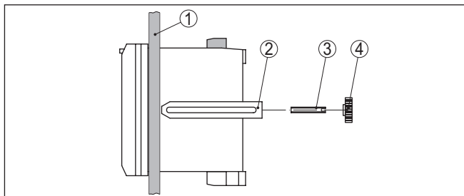
Рис. 2: Монтаж на панели
