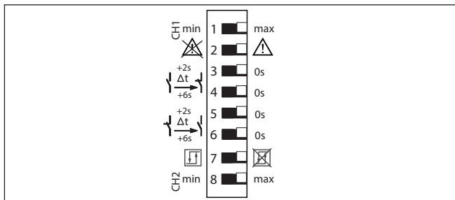
Рис. 3: DIL-переключатель VEGATOR 122
