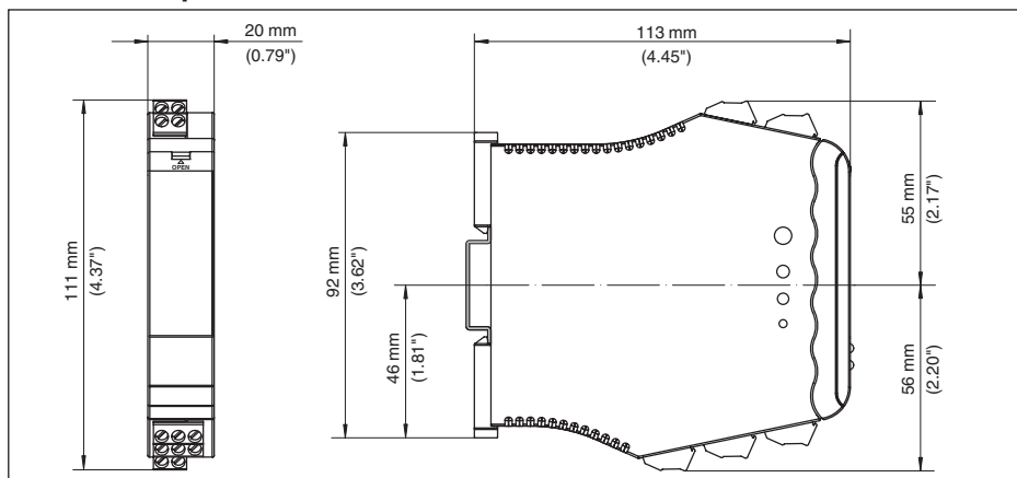
Рис. 54: Размеры VEGATOR 122
